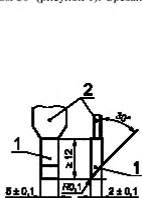
1 — платиновый электрод; 2 — медный удлинитель; 3 — опора; 4 — конец капелецницы; 5 — образец
