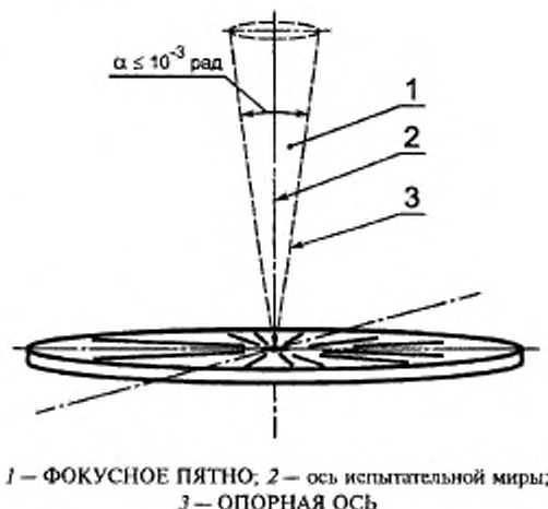
Рисунок 8 — Центрирование КАМЕРЫ ЗВЕЗДООБРАЗНОГО ИЗОБРАЖЕНИЯ
