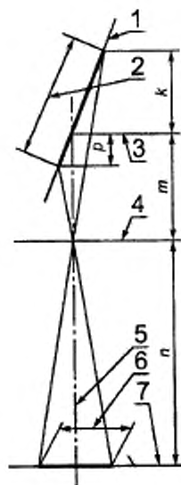
1 — плоскость АНОДА; 2 — длина ДЕЙСТВИТЕЛЬНОГО ФОКУСНОГО ПЯТНА; 3 — ОПОРНАЯ ПЛОСКОСТЬ; 4 — входная плоскость диафрагмы; 5 — ОПОРНАЯ ОСЬ; 6 — длина ЭФФЕКТИВНОГО ФОКУСНОГО ПЯТНА; 7 — РЕНТГЕНОГРАФИЧЕСКАЯ ПЛЕНКА
