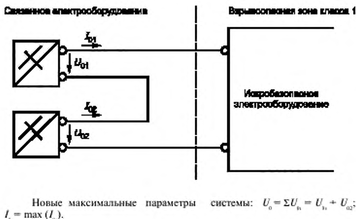
Рисунок В.1 — Последовательное соединение. Суммирование напряжений
