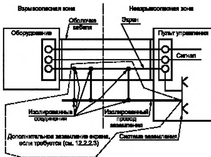
Рисунок 2 — Заземление проводящих экранов
