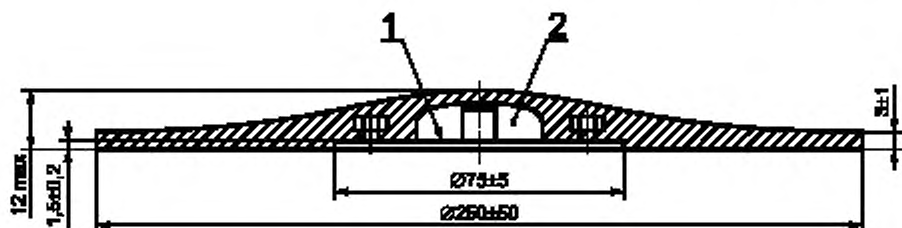
1 — тонкий металлический диск для установки акселерометра; 2 — полость для установки акселерометра
