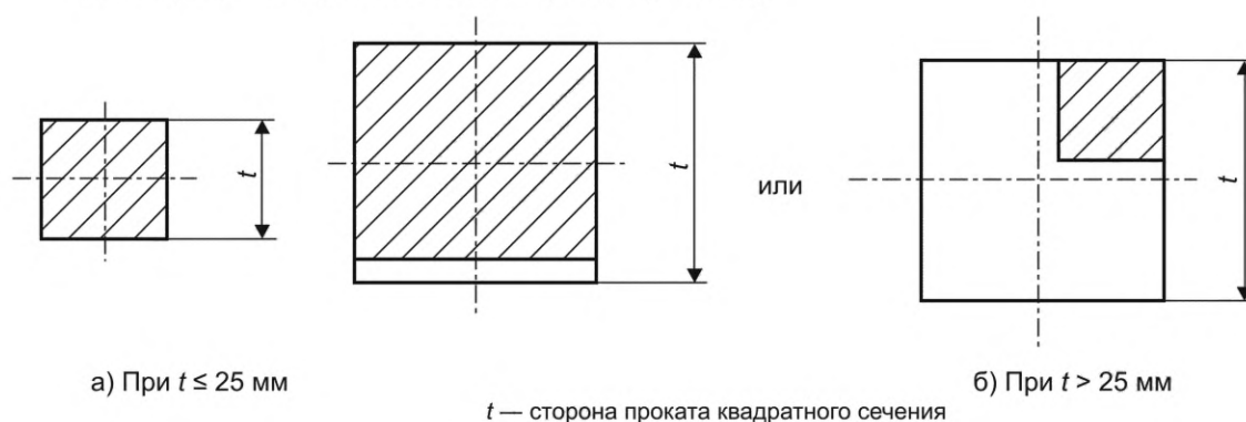
Рисунок В.2 — Схема отбора проб от проката квадратного сечения
