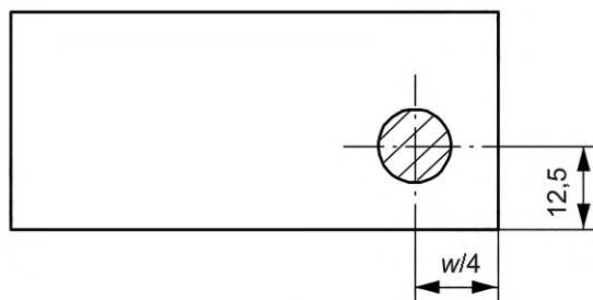
е) Цилиндрический образец при w > 50 мм и t \leq 50 мм
