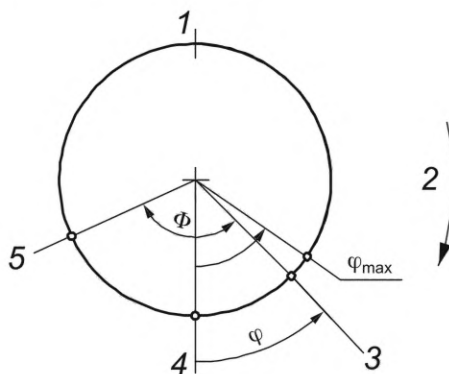
1 — TDC; 2 — направление вращения; 3 — сигнал подавления; 4 — BDC; 5 — сигнал остановки; \Phi — угол подавления (угол между сигналом подавления и сигналом остановки); \varphi — часть угла подавления до BDC, которая зависит от длины хода и положения поворотных кулачков и вычисляется как отрицательное значение после BDC; \varphi_{\max} — максимально допустимая часть угла подавления до BDC в градусах, вычисляемая из общей эффективности остановки системы и скорости, как описано далее
