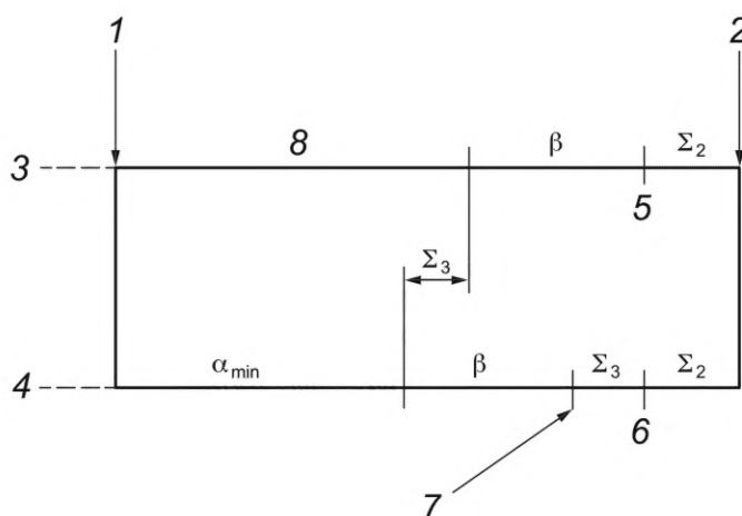
1 — сигнал остановки; 2 — контроль эффективности остановки; 3 — рабочее давление; 4 — минимальное давление; 5 — TDC; 6 — BDC; 7 — точка остановки при минимальном давлении; 8 — \alpha при рабочем давлении
