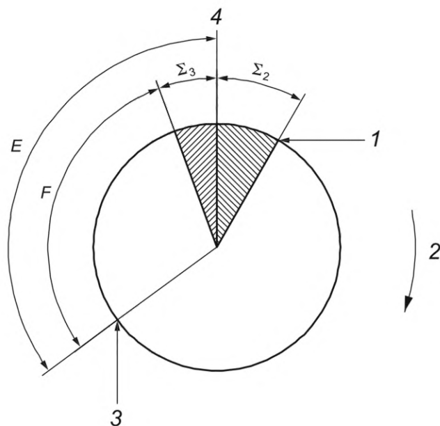
1 — контроль эффективности остановки; 2 — направление вращения; 3 — сигнал остановки; 4 — TDC; E — угол при рабочем давлении; F — угол при минимальном давлении
