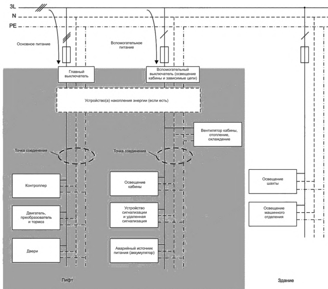
Рисунок А.1 — Подключение средств измерения энергопотребления лифтов
