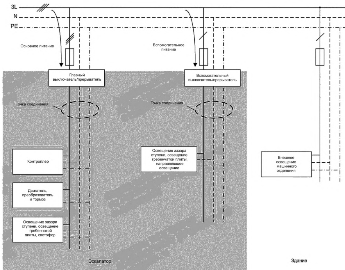
Рисунок А.2 — Подключение средств измерения энергопотребления эскалаторов
