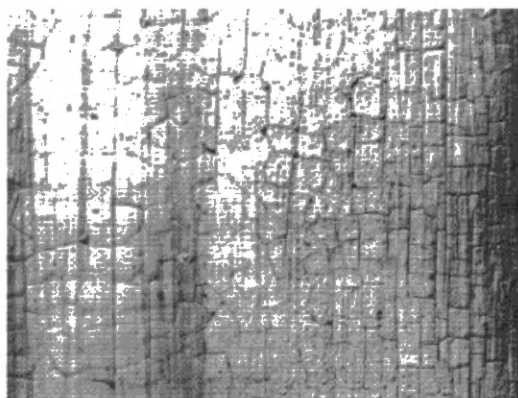
Рисунок 4 — Образование трещин «крокодиловая кожа»
