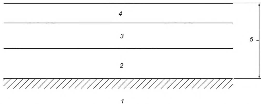
1 — окрашиваемая поверхность; 2 — лакокрасочное покрытие А; 3 — лакокрасочное покрытие В; 4 — лакокрасочное покрытие С; 5 — лакокрасочная система*
