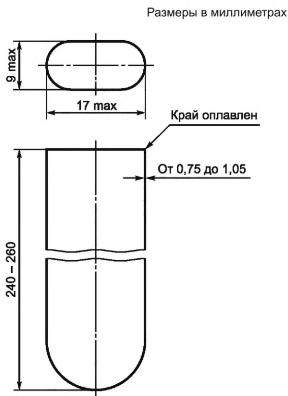
Рисунок 3 — Пробирка для осмотра и хранения пластинок
