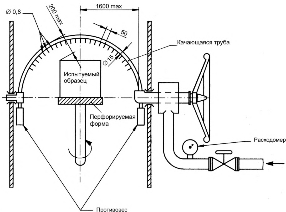
Рисунок 3 — Оборудование для испытаний на проникновение воды
