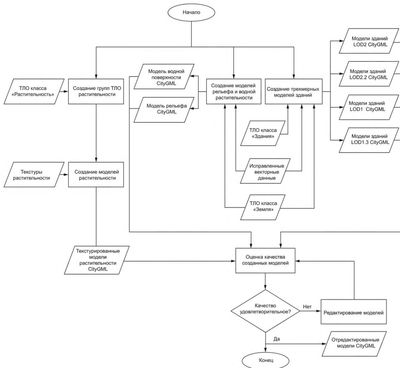
Рисунок А.8 — Трехмерное объектное моделирование объектов местности, технологическая схема создания объектных ЦПММ
