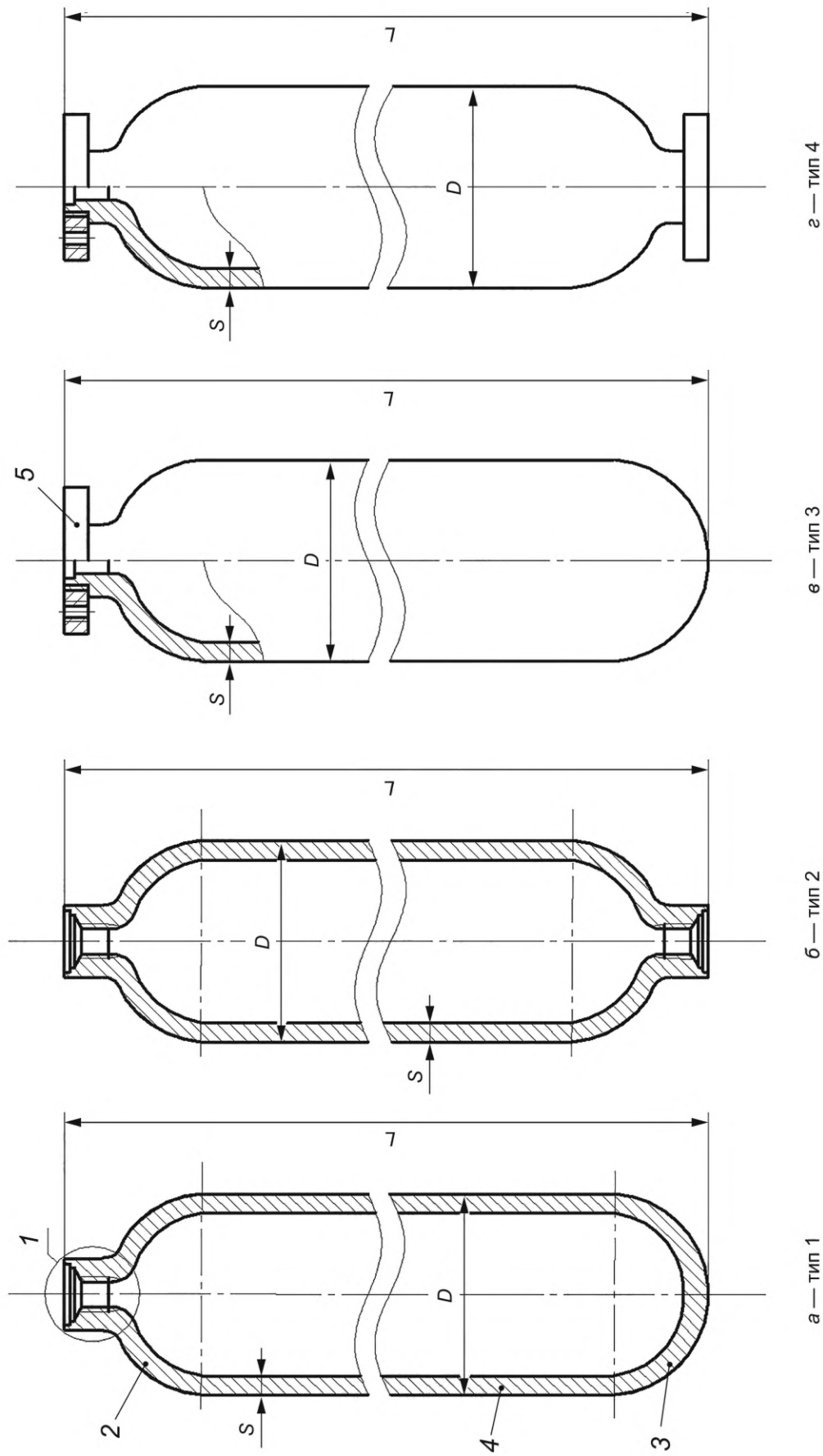
1 — горловина; 2 — днище с горловиной; 3 — глухое днище; 4 — цилиндрическая часть баллона; 5 — фланец; D — номинальный наружный диаметр цилиндрической части баллона; L — номинальная длина баллона; S — минимальная исполнительная толщина стенки цилиндрической части баллона
