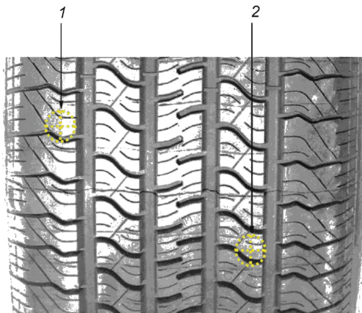
1 — точка измерений на внешнем ребре; 2 — точка измерений на внутреннем центральном ребре
