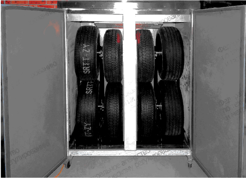
Рисунок В.1 — Пример специального стэнда для хранения шин (колес в сборе) Р1 и Н1 в холодильном шкафу
