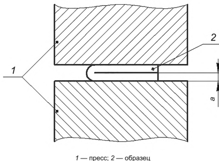
Рисунок 7 — Устройство для испытания образцов в виде продольных полос (сегментов)/поперечных полос до соприкосновения сторон образца
