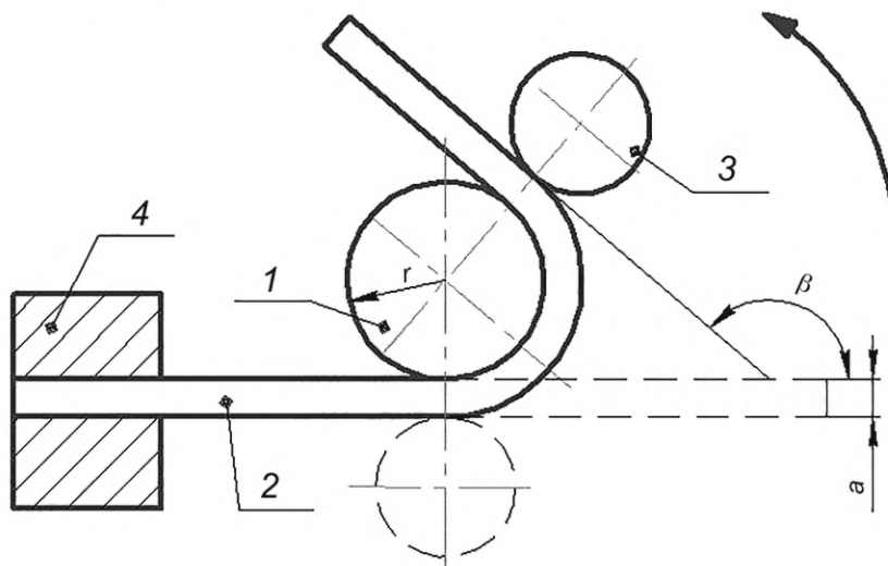
1 — оправка; 2 — образец; 3 — ролик; 4 — зажимное приспособление
