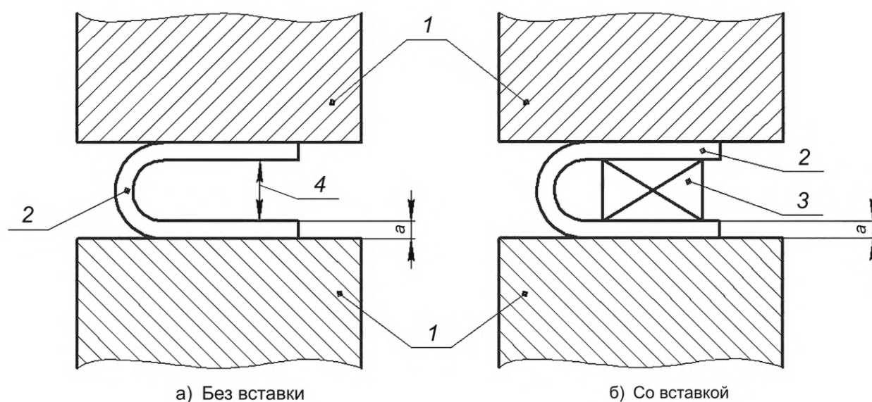
Рисунок 6 — Устройство для испытания образцов в виде продольных полос (сегментов)/поперечных полос до параллельности сторон
