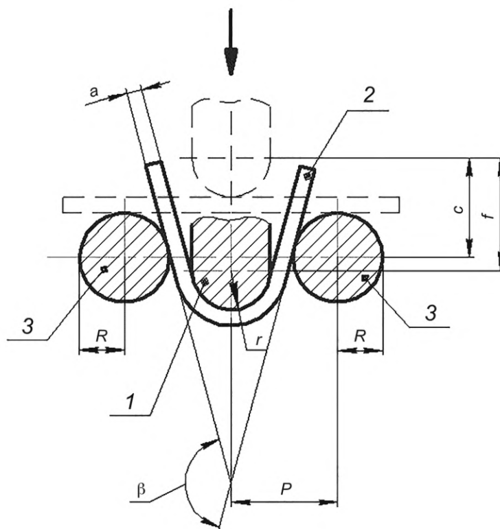
Рисунок А.1 — Параметры для расчета угла изгиба (загиба) \beta
