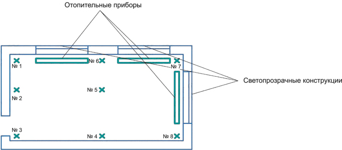
Рисунок А.2 — Потенциальные места установки датчика температуры в угловом помещении с тремя окнами
