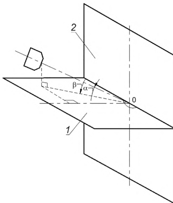
1 — горизонтальная плоскость; 2 — вертикальная плоскость; \alpha = 0^\circ (горизонтальный поток воздуха), +30^\circ и -30^\circ ; \beta = 0^\circ (скользящий поток воздуха), 15^\circ , 30^\circ , 45^\circ , 60^\circ , 75^\circ , 90^\circ (перпендикулярно к испытательной стенке)
