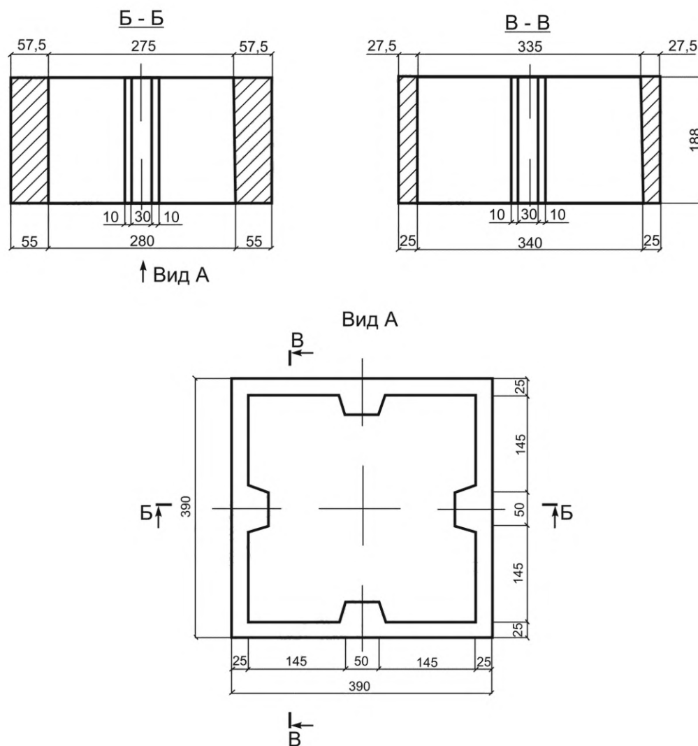
Рисунок А.21 — Камень для дымовой трубы
