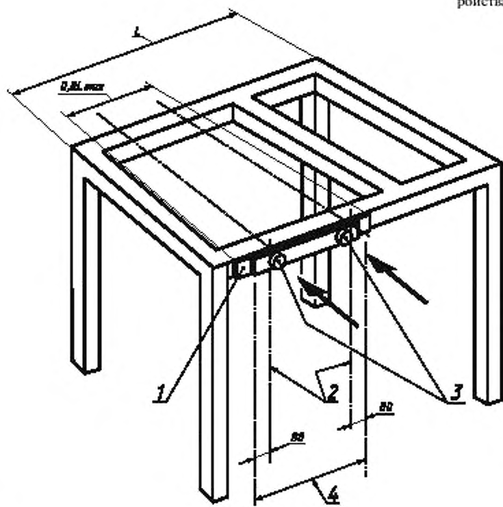
Рисунок 4 — Точка приложения боковой нагрузки к четырехъярусному ROPS
