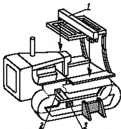
1 — балка для вертикального нагружения; 2 — заблокировано для предотвращения перемещения; 3 — блокировка противоположных трактов гусениц
