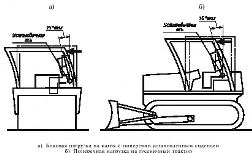
Рисунок 15 — Допускаемое вращение верхней части DLV относительно установочной оси
