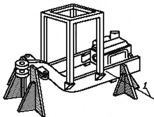
Рисунок 9 — Закрепление полурамы шарнирно-сочлененной машины
