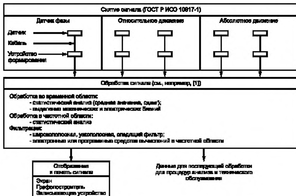
Рисунок 1 — Структура системы измерений вибрации вала
