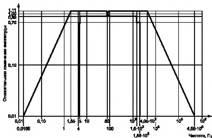
б) Рабочий диапазон частот от 5 до 1500 Гц
