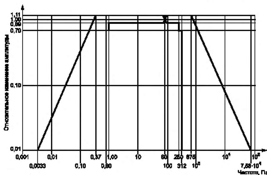
а) Рабочий диапазон частот от 1 до 250 Гц
