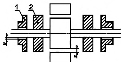
а — радиальный зазор между ротором и статором; g — радиальное перемещение, допускаемое подшипниковым щитом; 1 — подшипниковый щит; 2 — подшипник скольжения
