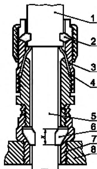
1 — внешняя оболочка кабеля; 2 — внешнее уплотнительное кольцо; 3 — крепящий зажим для брони; 4 — броня; 5 — оболочка внутреннего; 6 — уплотнительное кольцо; 7 — резьбовой ввод; 8 — стенка оболочки; x — осевая высота уплотнительного кольца
