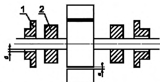
а — радиальный зазор между статором и ротором; g — допустимое изменение радиального зазора в подшипниковом щите; 1 — подшипниковый щит; 2 — подшипник скольжения
