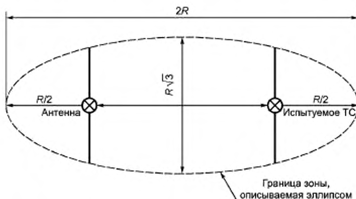
Рисунок В.1 — Зона измерительной площадки с поворотной платформой, свободная от предметов, отражающих электромагнитную энергию
