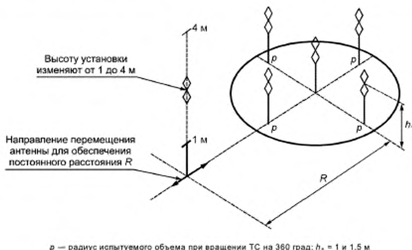
Рисунок Д.1 — Расположения антенн при измерении затухания альтернативной площадки (вертикальная поляризация)
