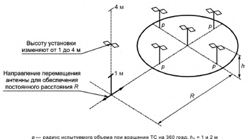
Рисунок Д.2 — Расположения антенн при измерении затухания альтернативной площадки (горизонтальная поляризация)
