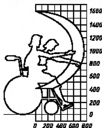
Рисунок Б.2 — Зона досягаемости для инвалидов-женщин в кресле-коляске
