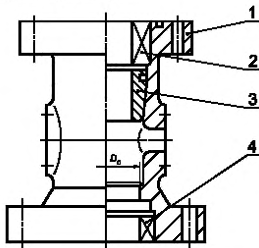
1 — корпус; 2 — верхний уплотнитель; 3 — трубо- держатель; 4 — нижний уплотнитель
