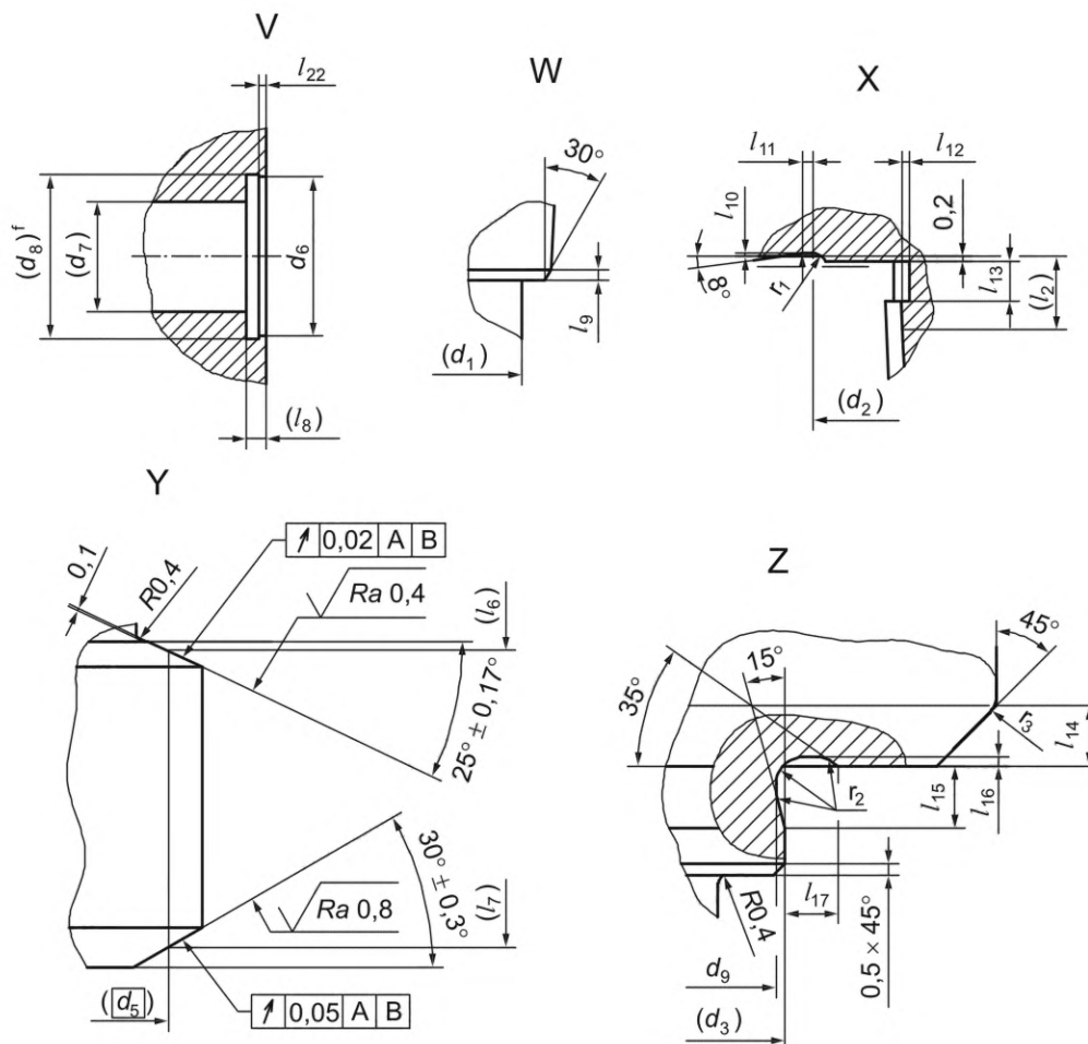
b) Элементы с основного вида хвостовика типа F
