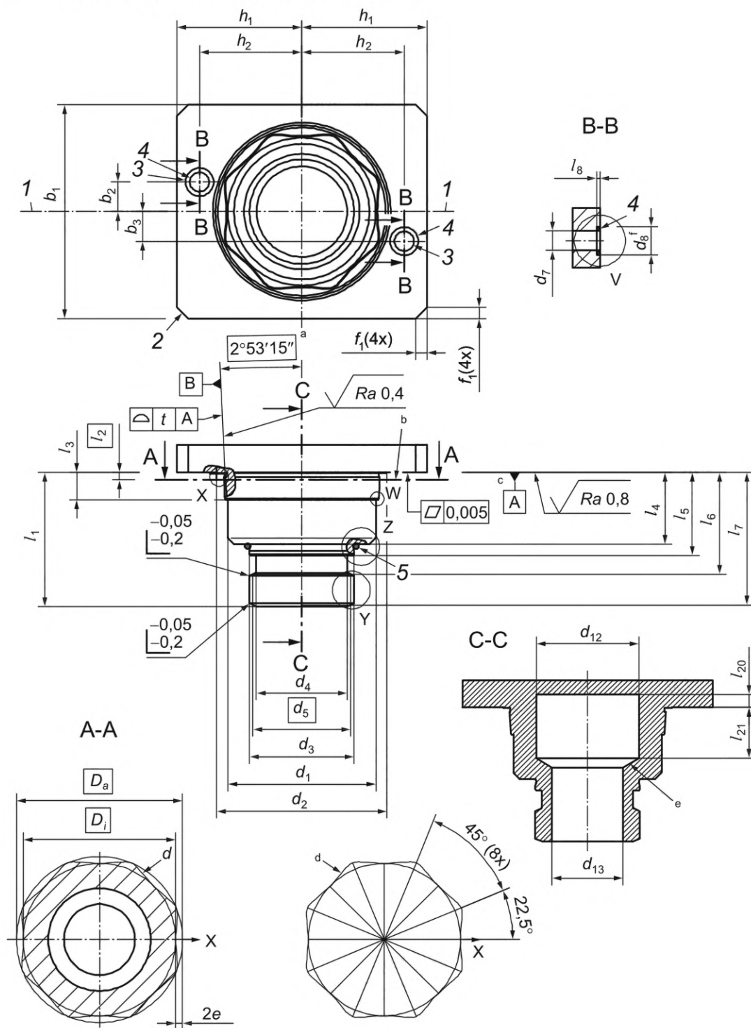
а) Общий вид хвостовика типа F
