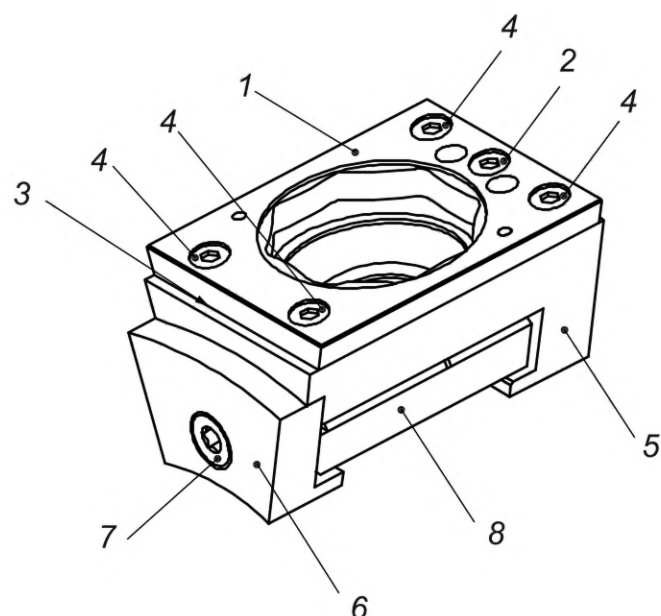
Рисунок D.2 — Возможный нестандартизованный вариант фланца с многоугольным посадочным гнездом
