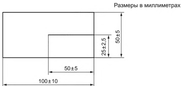
Рисунок 3 — Размеры испытываемой пробы
