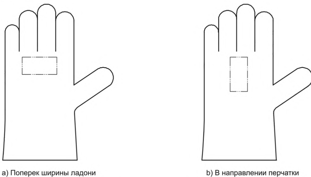
Рисунок 5 — Испытание на раздир. Испытуемые области
