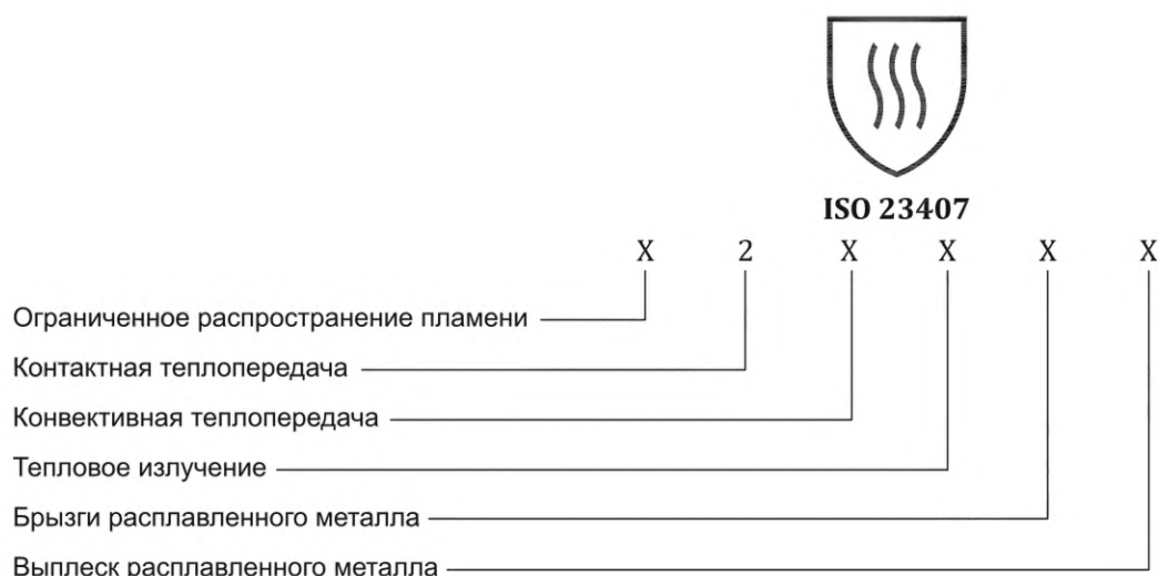
Рисунок 9 — Пример маркировки без ограниченного распространения пламени
