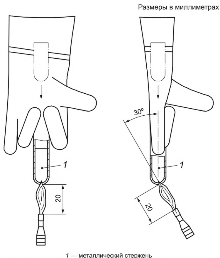
Рисунок 2 — Установка испытуемой перчатки (имитатор пальца)
