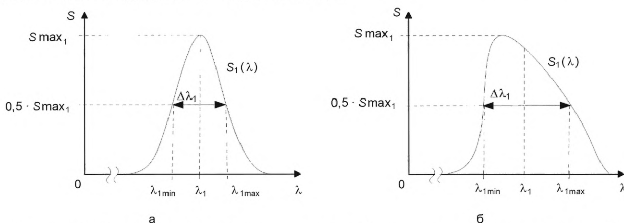
Рисунок А.1 — Примеры зависимостей чувствительности S_1(\lambda) в спектральных каналах симметричной (а) и несимметричной (б) формы. Площади под кривой S_1(\lambda) слева и справа от \lambda_1 равны
