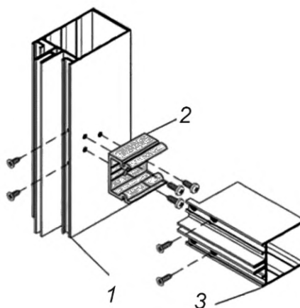
1 — стойка; 2 — сухой соединитель (закладной элемент); 3 — ригель
