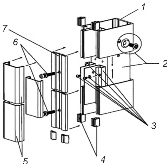
1 — стойка; 2 — сухой соединитель (закладной элемент); 3 — крепежные изделия; 4 — уплотнитель; 5 — декоративная планка стойки; 6 — винт; 7 — прижимная планка
