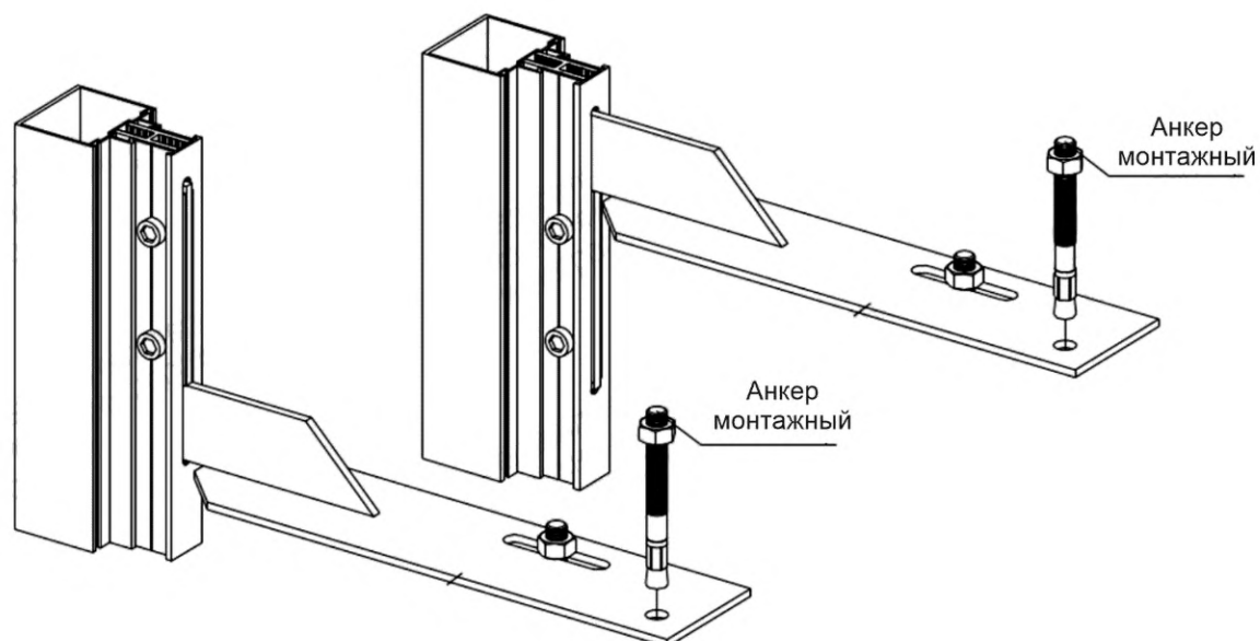
Рисунок Д.7 — Крепление с применением стальных кронштейнов с сухарным соединителем (закладным элементом) под метрическую резьбу, установленным на стойку в процессе сборки
