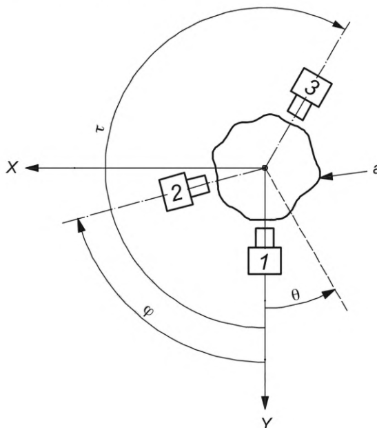
с 1—3 — датчики; \theta — угол, измеренный от оси Y; \tau — угол между датчиком 1 и датчиком 3; \varphi — угол между датчиком 1 и датчиком 2; a — профиль округлости
