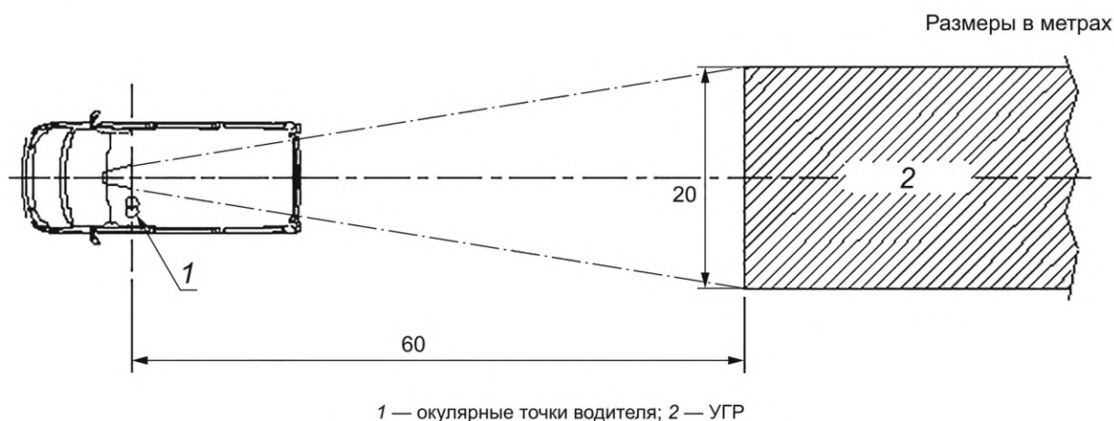
Рисунок 8 — Поле обзора устройства класса I
