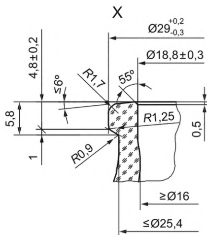
д) Модель С: бутылка для инфузионных растворов с горловиной 29 мм
