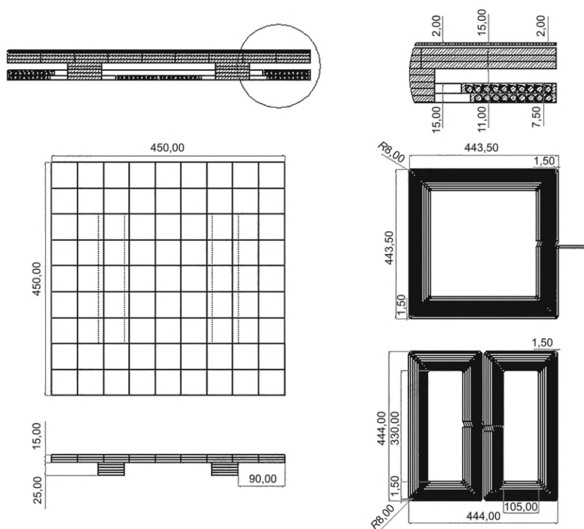
Рисунок В.5 — Размеры эталонного принимающего устройства MF-WPT4/Z2
