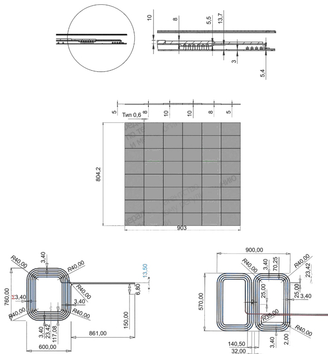
Рисунок А.8 — Размеры эталонного принимающего устройства MF-WPT4/Z3
