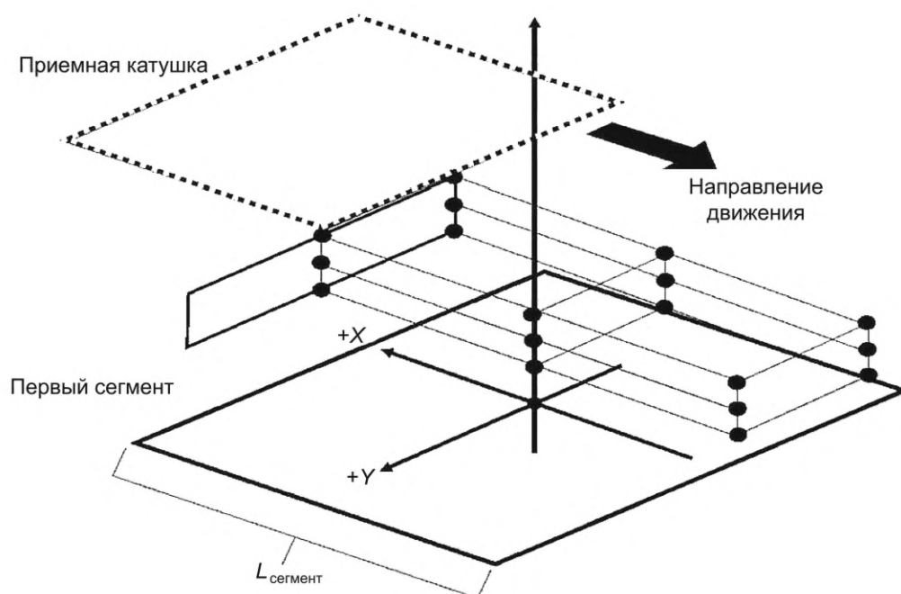
Рисунок 4 — Измерение эффективности D-WPT
