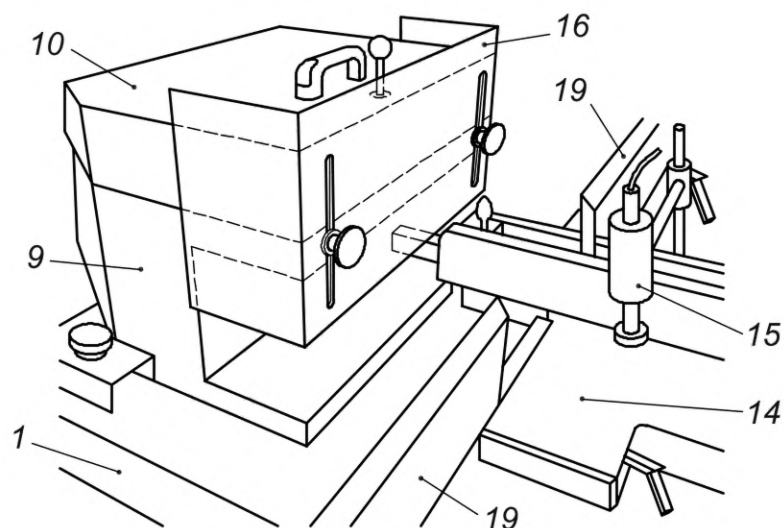
с) пример защиты инструмента для шипорезных работ с фиксированными и регулируемыми защитными кожухами, установленными на станке и на подвижном столе
