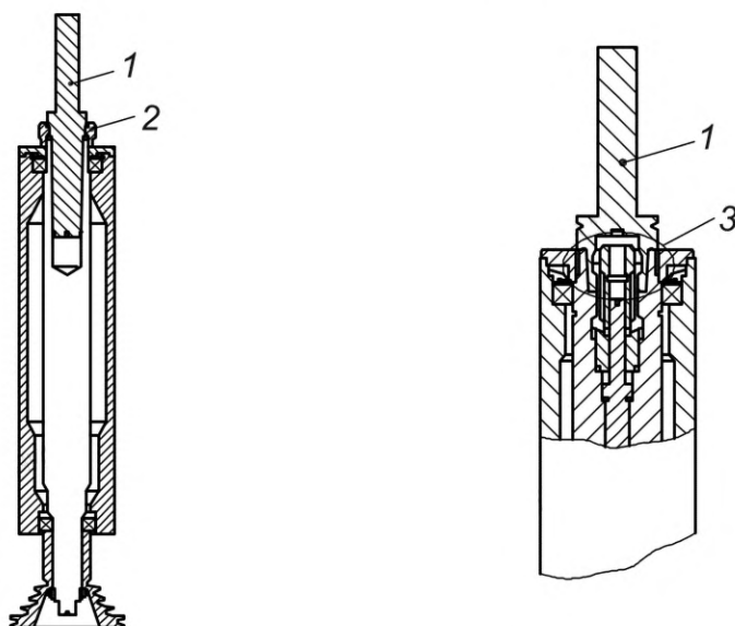
а) съёмная оправка
