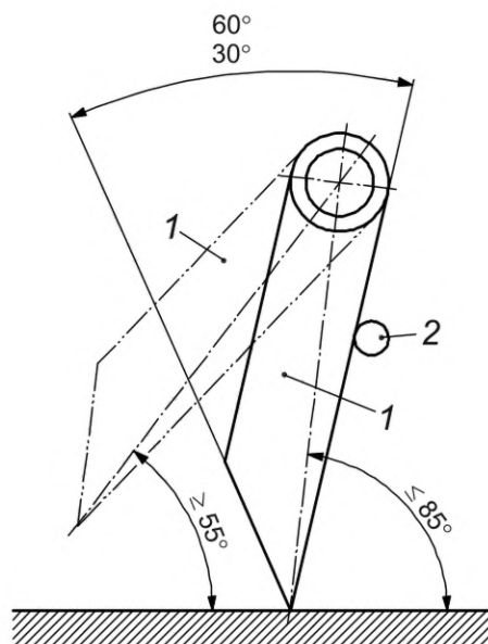
1 — противоосколочный палец; 2 — механический концевой упор
