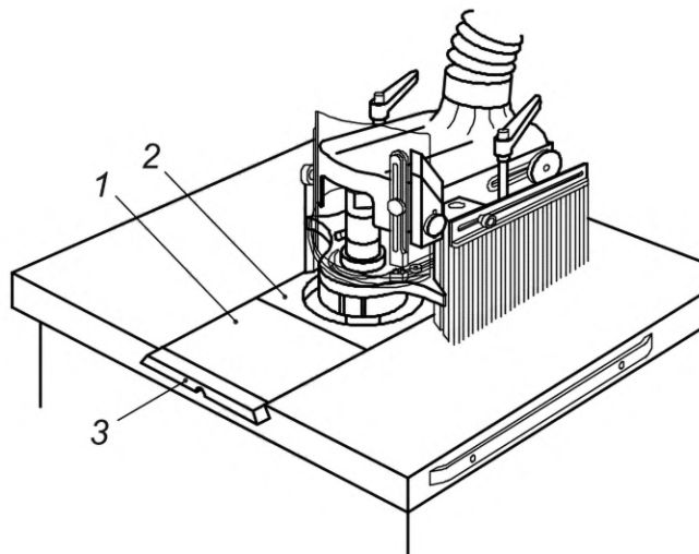
1 — регулируемая вставка стола; 2 — легко обрабатываемая часть вставки стола; 3 — мягкая материальная часть вставки стола
