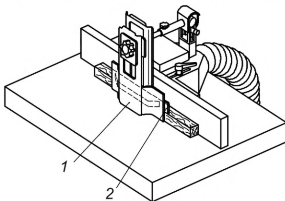
1 — прижимная защитная накладка; 2 — планка прижима к столу
