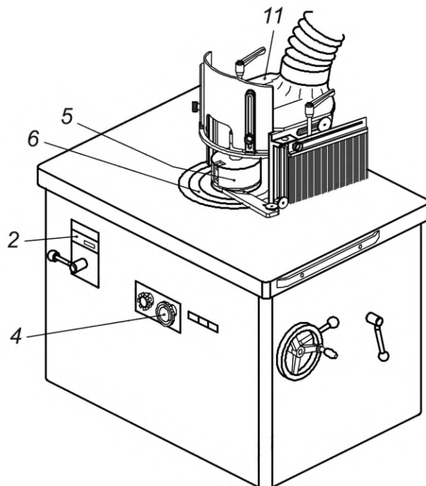
б) пример фрезерного вертикального станка с нижним расположением шпинделя, оборудованного для криволинейной обработки
