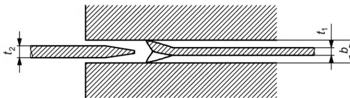
Рисунок 12 — Толщина пластинчатого разделителя в зависимости от размеров дисковой пилы
