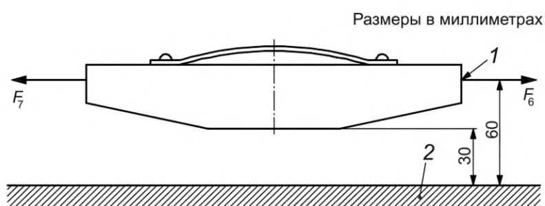
Рисунок Н.4 — Точки измерения прогиба накладки прижима к столу и направления приложения испытательных сил — Вид сбоку*
