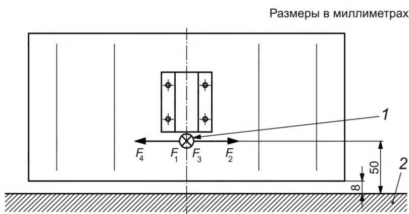
Рисунок Н.1 — Точки измерения прогиба прижимной защитной накладки и направлений приложения испытательных усилий — Вид сбоку*
