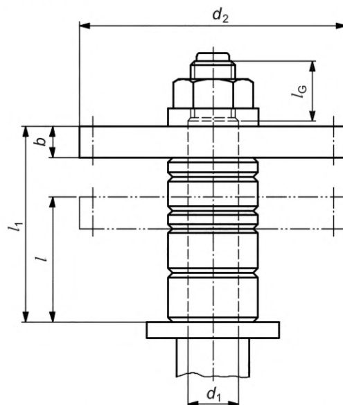
Рисунок G.1 — Иллюстрация размеров оправки
