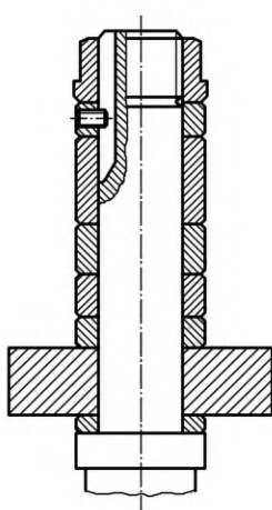
а) Пример оправочной гайки
