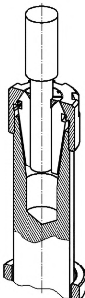
с) Пример оправки для инструмента с хвостовиком
