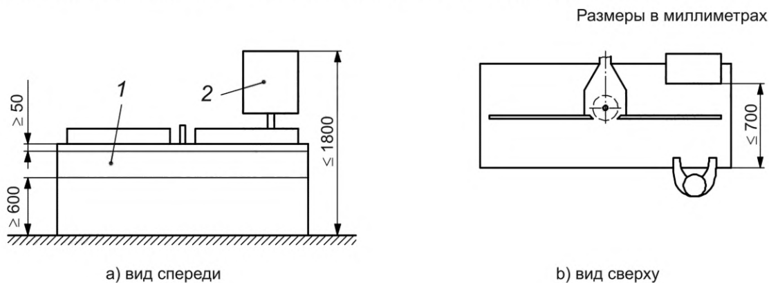
Рисунок 8 — Положение органов управления
