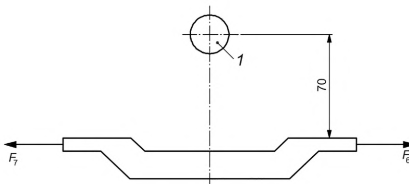
Рисунок Н.5 — Точки измерения прогиба накладки прижима к столу и направления приложения испытательных сил - Вид сверху
