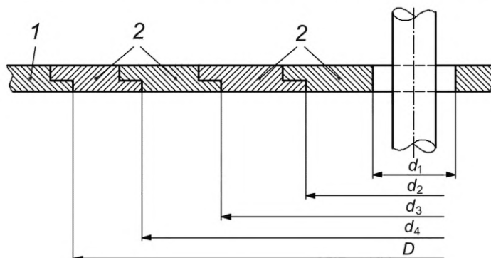
Рисунок 16 — Кольца стола
