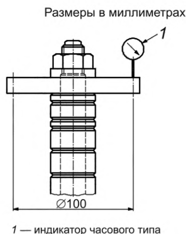
Рисунок 10 — Комплект оправочных колец, конфигурация для испытания на осевое биение
