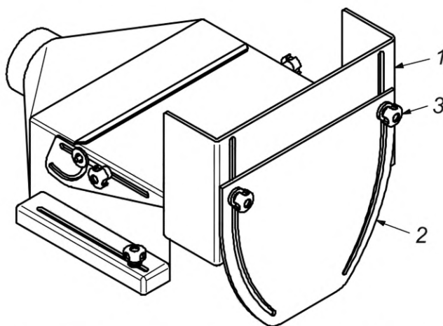
1 — регулируемый вручную защитный кожух; 2 — саморегулирующееся ограждение; 3 — устройство с двойной функцией: для регулировки детали № 1 и направляющей детали № 2
