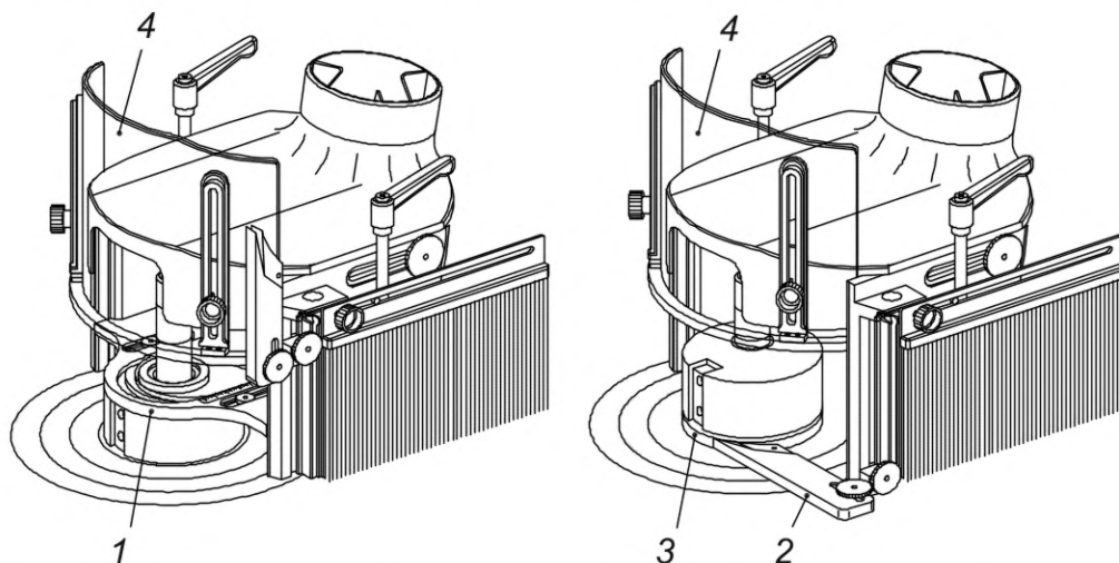
1 — полукруглая направляющая; 2 — вводное устройство для крепления заготовки с шаблоном; 3 — копирное кольцо (наружное кольцо шарикоподшипника); 4 — перемещаемое ограждение (щиток защиты рук)
