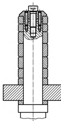
б) Пример оправочного винта
