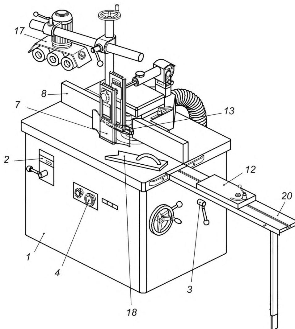
а) пример фрезерного вертикального станка с нижним расположением шпинделя, оборудованного для прямолинейной обработки;
