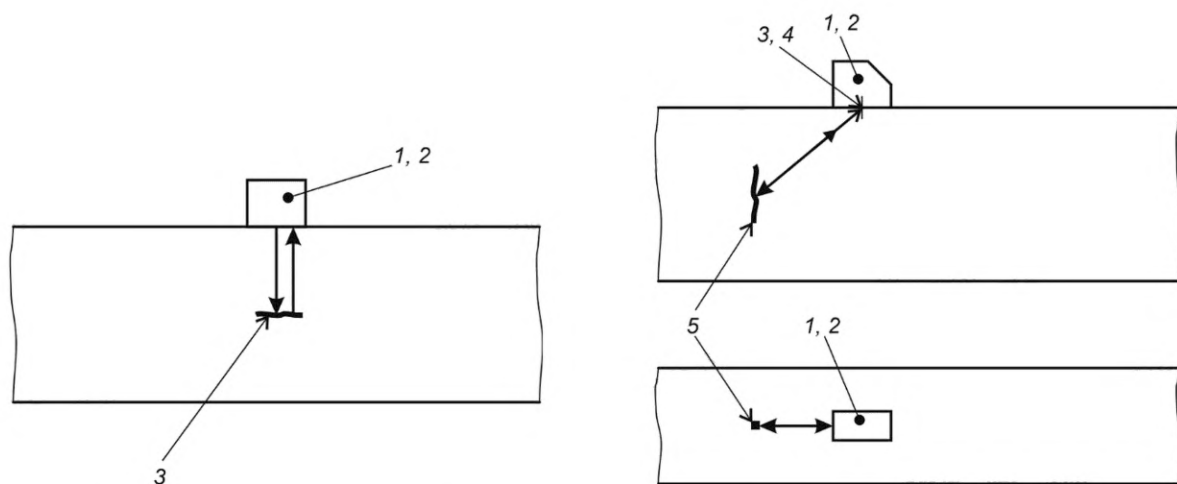
а) схема контроля эхо-методом с использованием совмещенного прямого преобразователя
