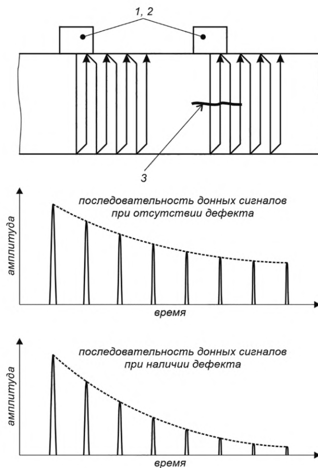
в) метод многократных отражений
