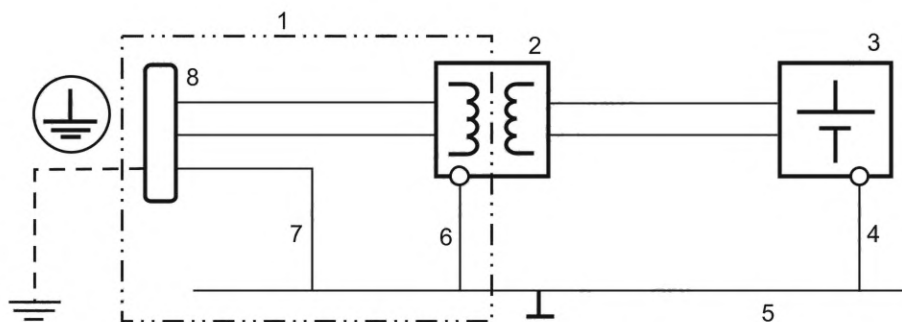
1 — цепь питания транспортного средства в соответствии с ИСО 5474-2; 2 — зарядное устройство с простым разделением; 3 — ПСХЭЭ; 4 — уравнивание потенциалов в соответствии с ИСО 6469-3; 5 — электрическое шасси; 6 — защитный проводник; 7 — защитный проводник; 8 — ввод транспортного средства
