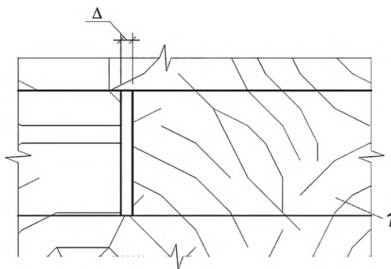
Рисунок Б.14 — Отклонения поверхности покрытия пола (промежуточных элементов пола) от плоскости
