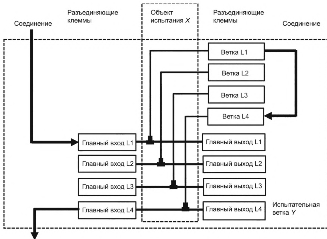
Рисунок Н.7 — Пример принципиальной схемы в случае испытаний ответвления четырехжильной кабельной соединительной гильзы на короткое замыкание от основной цепи к ответвлению через соседние фазы L4—L1 с противоположным протеканием тока
