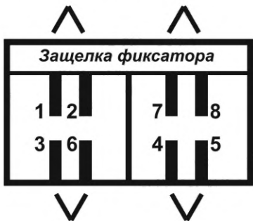
Рисунок 10 — Раскладка проводов отдельных пар по контактам розетки (см. [63]) категорий 7, 7 A , 8.2 и BNC-B
