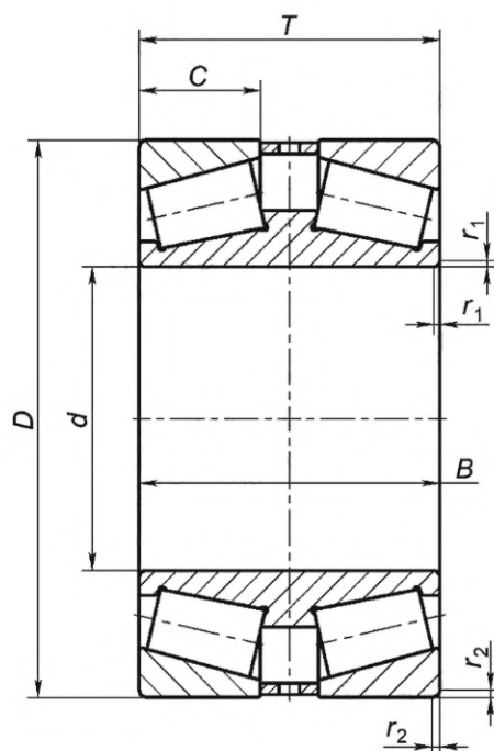
Рисунок 3 — Конструктивное исполнение 84
