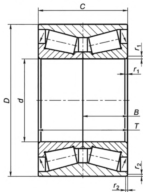
Рисунок 2 — Конструктивное исполнение 53
