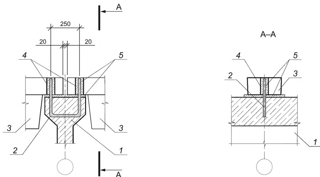
1 — балка стропильная; 2 — закладная деталь балки; 3 — прогон; 4 — закладная деталь прогона; 5 — участки конструкции, заполняемые раствором
