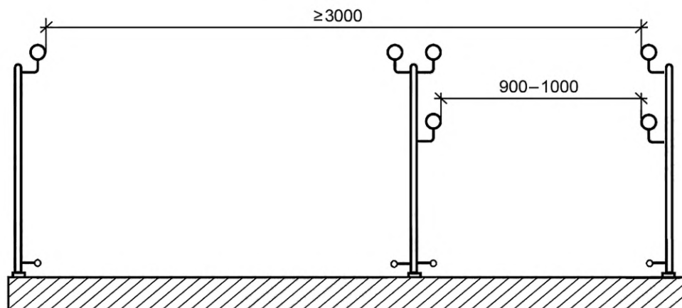
Рисунок 7 — Расположение поручней на пандусе шириной более 3 м
