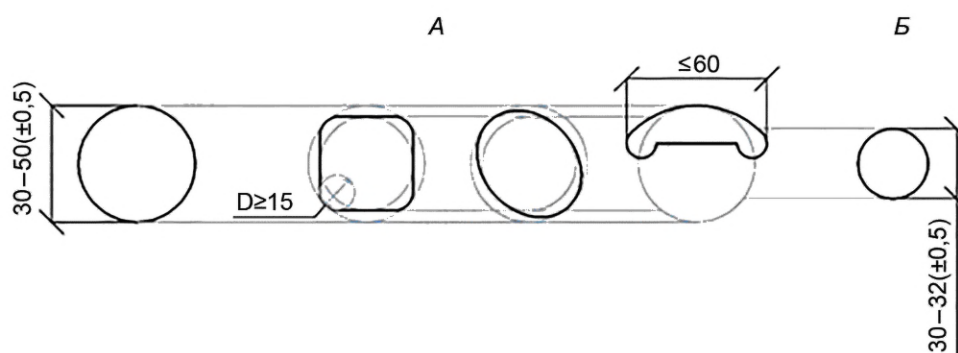
А — поручни для взрослых пользователей; Б — поручни для детей
