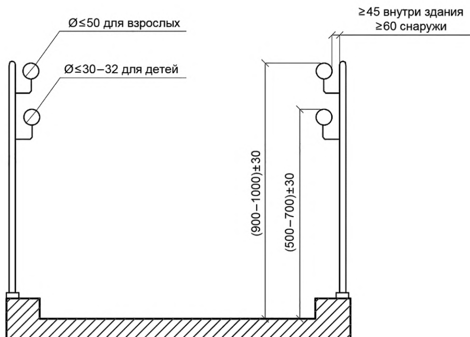
Рисунок 17 — Поручни на горизонтальных путях движения
