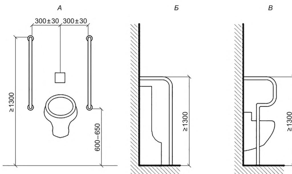
А — поручни настенного крепления у писсуара; Б, В — поручни напольно-настенного крепления
