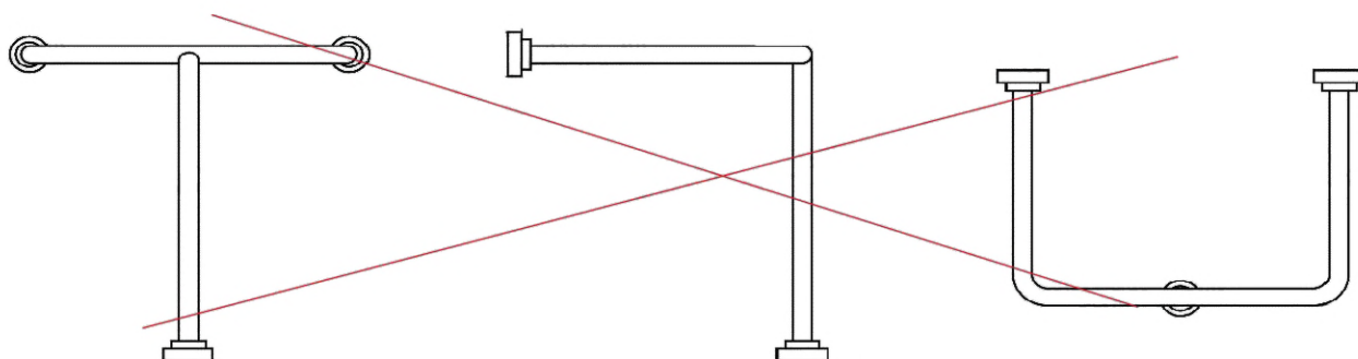
Рисунок А.12 — Недопустимая конструкция поручня у раковины с опорой по центру
