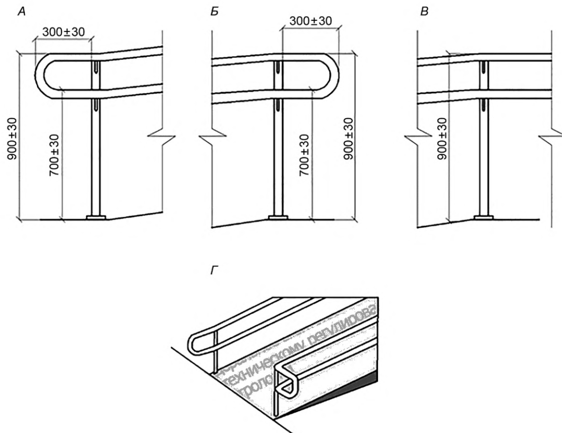
А — горизонтальные завершения поручня на нижней площадке; Б — горизонтальные завершения поручней на верхней площадке; В — поручни пандуса, переходящие в ограждение горизонтальной площадки; Г — горизонтальные завершения поручней на пандусе в стесненных условиях
