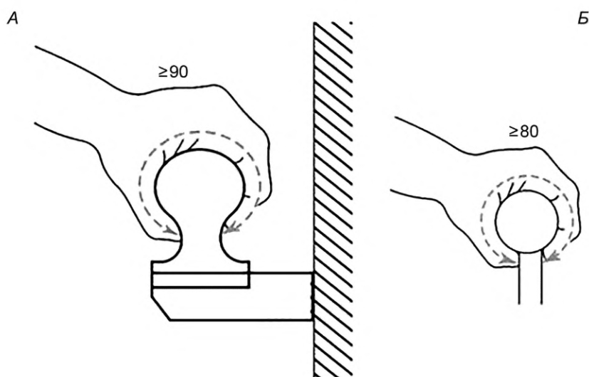
А — поручни для взрослых пользователей; Б — поручни для детей
