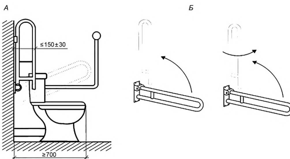
А — допустимая ширина откидного поручня, размещенного в зоне пересадки с кресла-коляски; Б — конструкция поручня с поворотно-откидным механизмом
