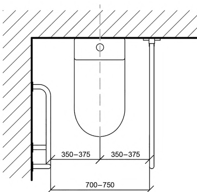
Рисунок 22 — Расстояние между поручнями у унитаза
