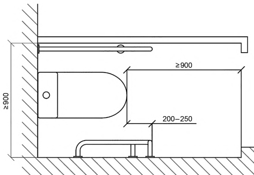
Рисунок 30 — Комбинированный поручень в адаптированной кабине уборной в блоке мужских и женских санитарно-бытовых помещений
