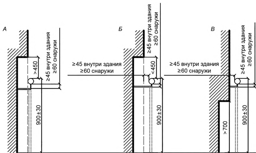
А — поручень под выступом, нависающем над поручнем на высоту более 450 мм; Б — поручень под выступом, нависающем над поручнем на высоту менее 450 мм; В — поручень перед выступом на высоте ниже крепления поручня
