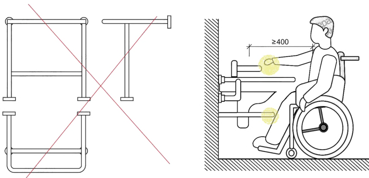
Рисунок А.14 — Поручень к раковине с нижней планкой для защиты слива затрудняет доступ к крану инвалиду, использующему кресло-коляску
