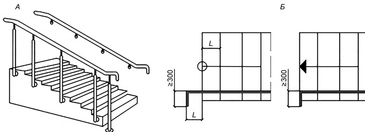
А — поручни лестниц; Б — поручни лестниц в стесненных условиях; L — ширина ступеней
