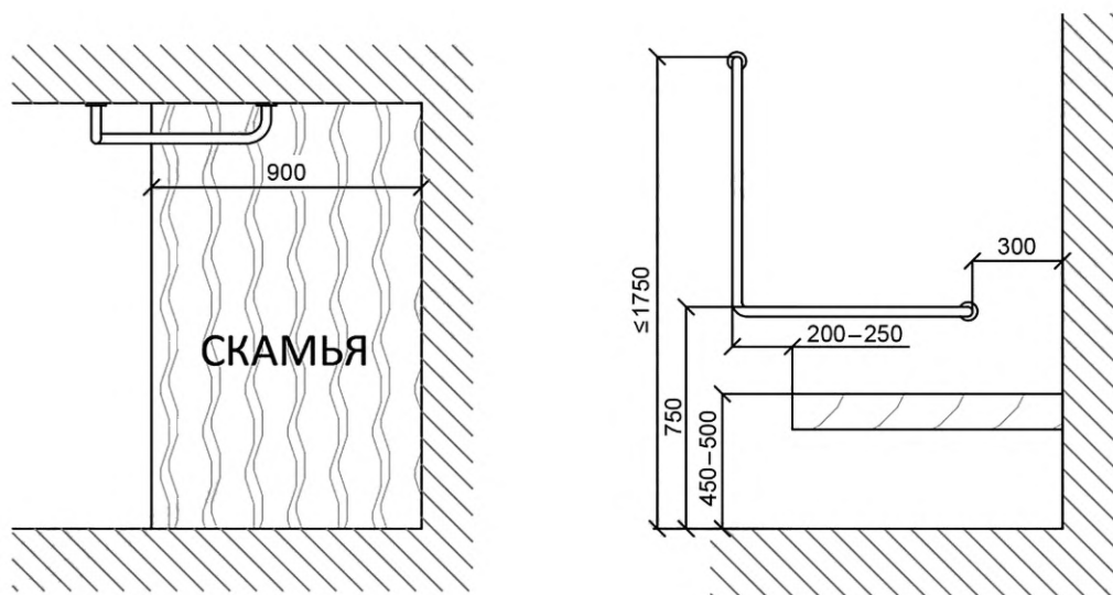
Рисунок 39 — Поручни в доступной примерочной кабине
