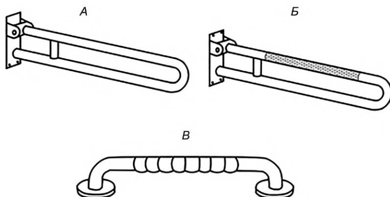
А — поручни из нержавеющей стали; Б — поручни с мелкой насечкой; В — поручни с рифлением поверхности ребрами с закруглением
