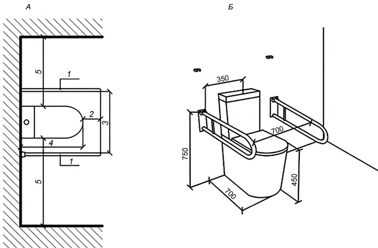
А — вид сверху; Б — объемное представление; 1 — откидной поручень; 2 — вынос поручня — не менее 150 мм; 3 — расстояние между поручнями от 700 до 750 мм; 4 — длина унитаза 700 мм; 5 — ширина зоны для размещения кресла-коляски \geq 800 мм (при реконструкции \geq 750 )
