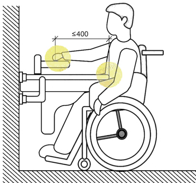
Рисунок А.11 — Расположение поручня по переднему краю раковины затрудняет доступ к крану инвалиду, использующему кресло-коляску
