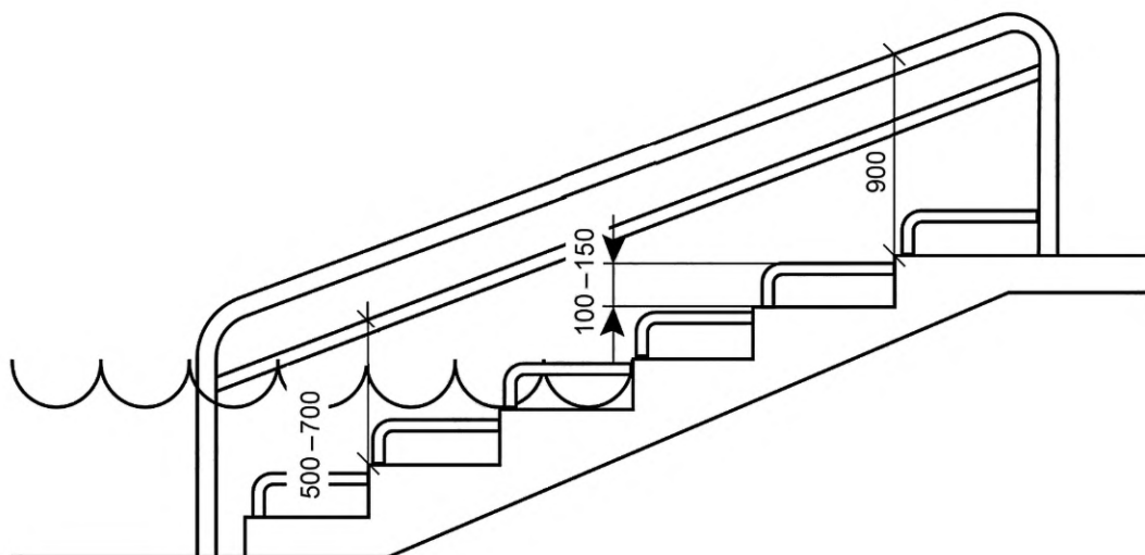
Рисунок 37 — Поручни на пологой лестнице в бассейн
