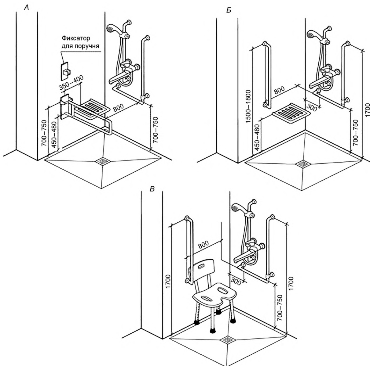
А — откидной и комбинированный поручни в душевой кабине; Б, В — вертикальный и комбинированный поручни в душевой кабине
