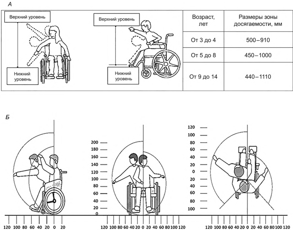
А — зона досягаемости для детей, использующих кресло-коляску; Б — для инвалидов, использующих кресло-коляску
