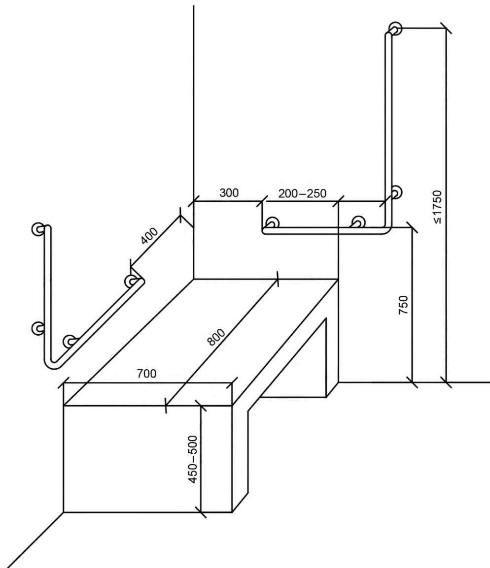
Рисунок 38 — Поручни у скамьи для переодевания
