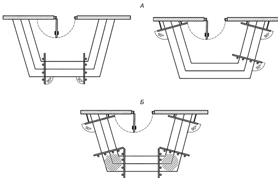
А — варианты расположения поручней на лестнице неправильной формы при центральном и боковом подходе; Б — недопустимый вариант расположения поручней с «тупиковыми» углами, опасными для незрячих пользователей
