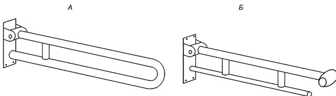
А — соединение концевых элементов поручня; Б — скругление концевых элементов
