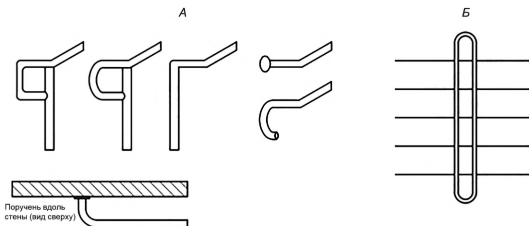
А — варианты завершающих частей поручней на лестницах; Б — окончания двухсторонних разделительных поручней
