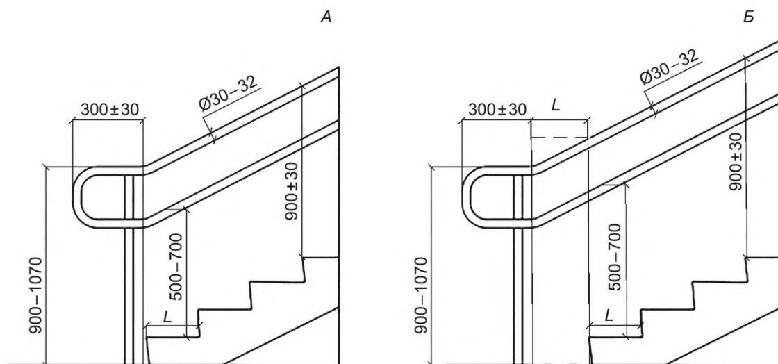
А — минимальный вылет завершающей горизонтальной части поручней; Б — оптимальный вылет завершающей части поручней с дополнительным наклонным участком на ширину ступени при отсутствии стесненных условий
