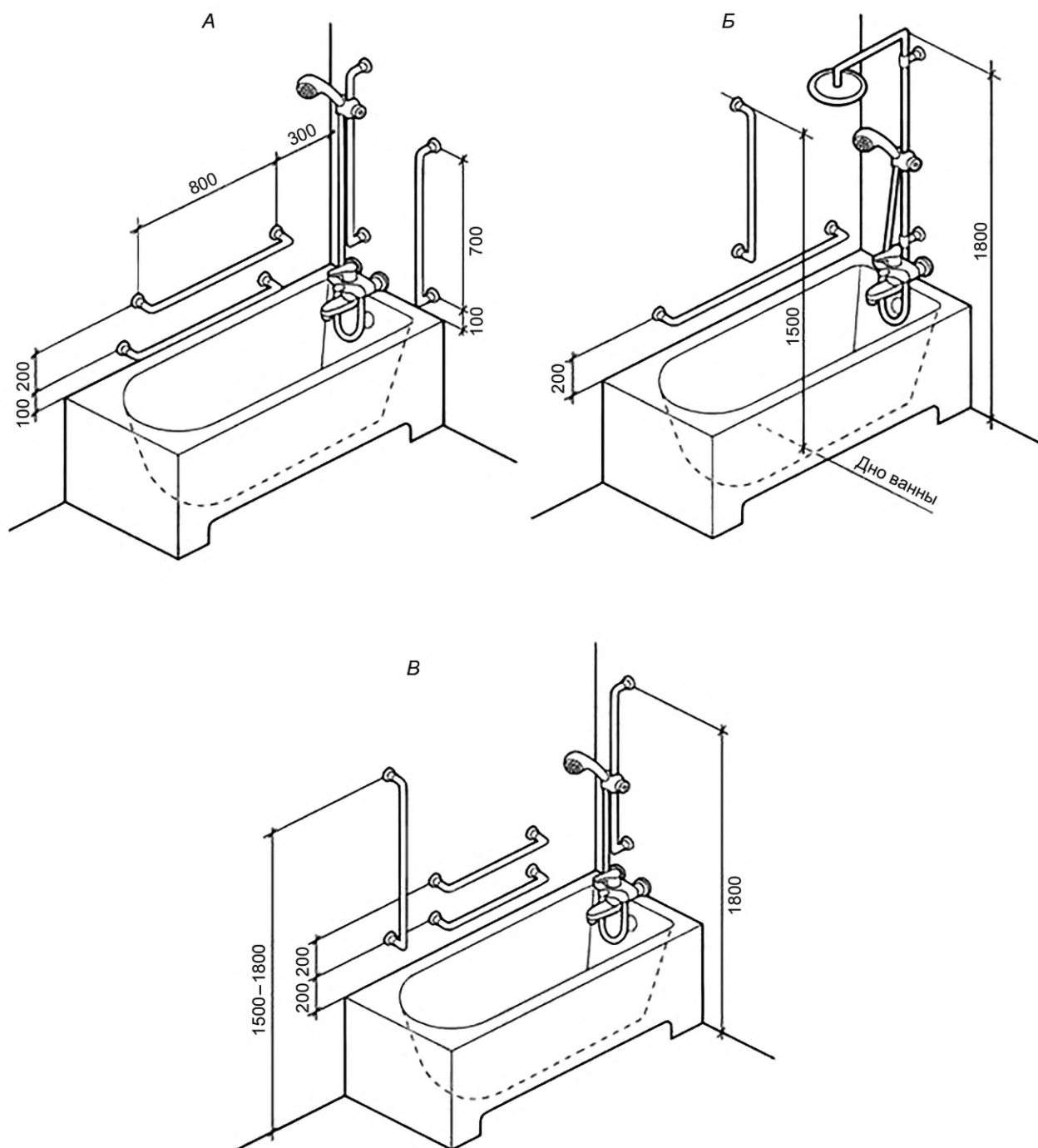
А — размещение двух уровней горизонтальных поручней вдоль длинного борта ванны и вертикального поручня перед ванной; Б — вертикальный и горизонтальный поручни вдоль длинного борта ванны; В — два уровня горизонтальных поручней и вертикальный поручень
