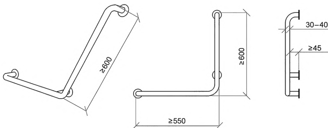
Рисунок 29 — Примеры конструкции комбинированных поручней
