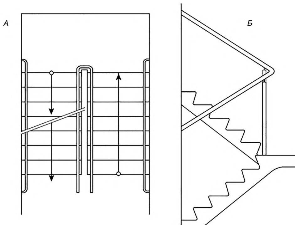
А — внешние и внутренние поручни на многомаршевой лестнице; Б — непрерывность внутреннего поручня многомаршевой лестницы
