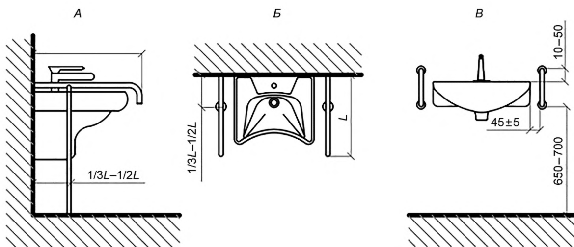
А — поручень настенно-напольного крепления с дополнительной вертикальной опорой, вид сбоку; Б — поручни настенно-напольного крепления с дополнительной вертикальной опорой, вид сверху; В — настенное крепление поручня
