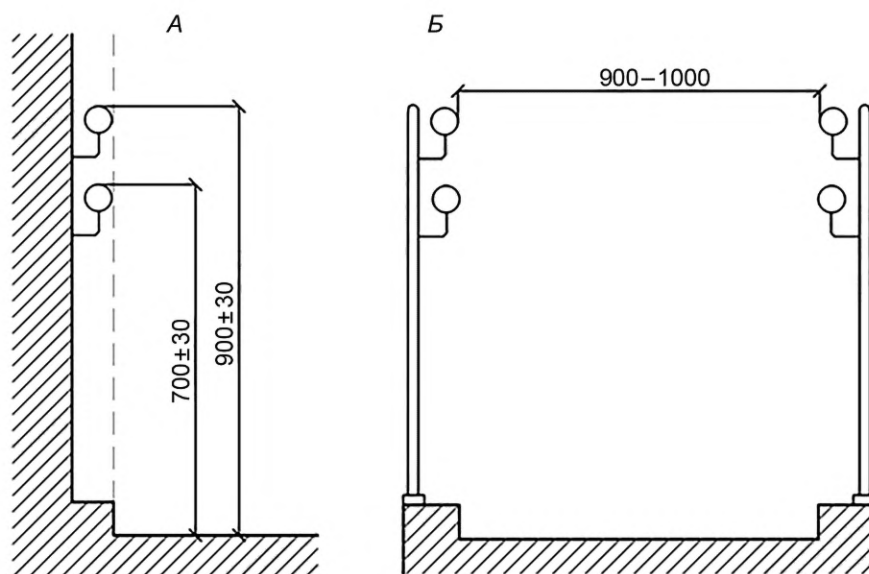
А — высота поручней; Б — расстояние между поручнями ограждений пандуса
