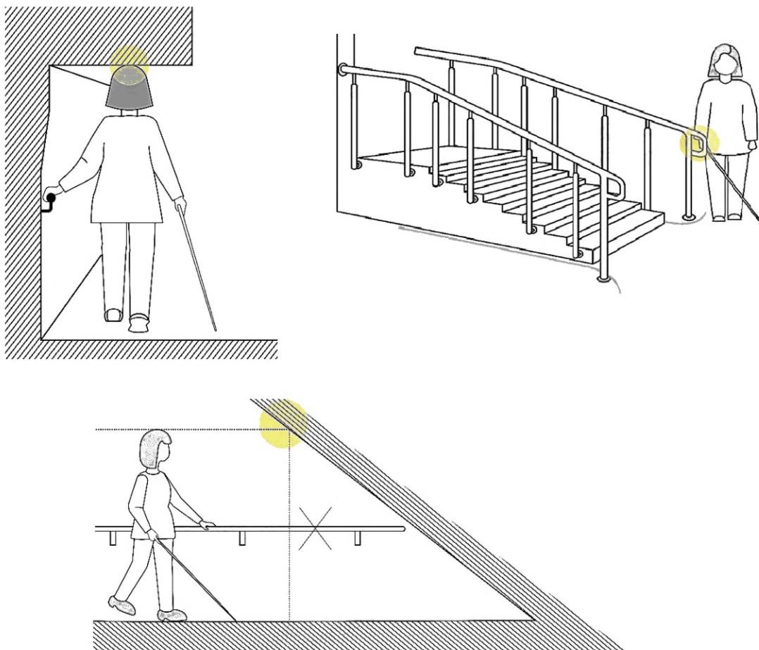
Рисунок А.4 — Расположение поручней, не обеспечивающее безопасность для незрячих пользователей
