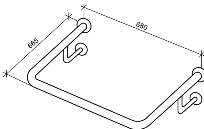
Рисунок А.13 — Конструкция и габариты поручня, затрудняющие доступ к крану инвалиду, использующему кресло-коляску
