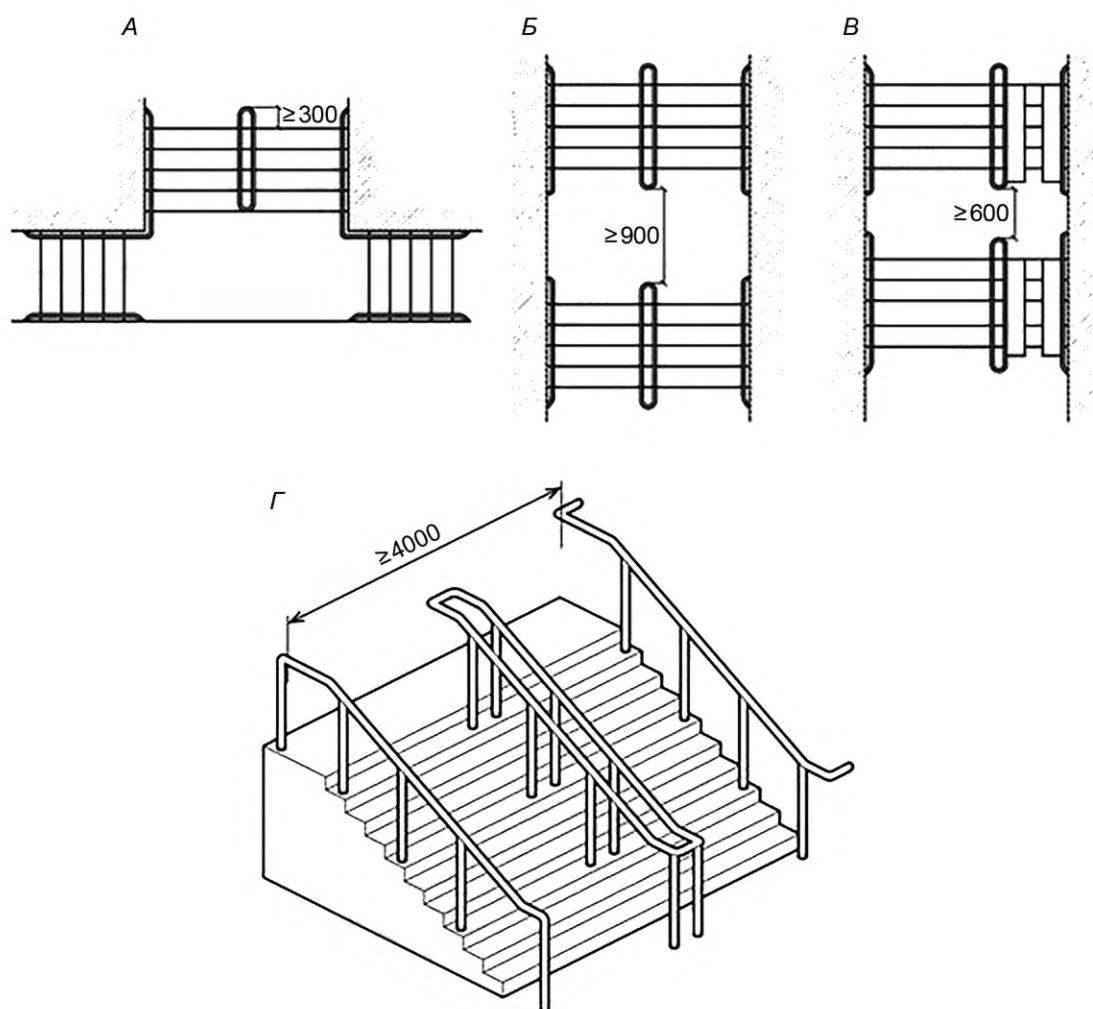
А, Б — поручни с двух сторон на открытых лестницах (расположенных вне лестничных клеток); В — с двух сторон и с разделительным поручнем на лестницах, имеющих колясочные спуски (аппарели); Г — с двух сторон и с центральным разделительным поручнем на лестницах, имеющих ширину более 4 м
