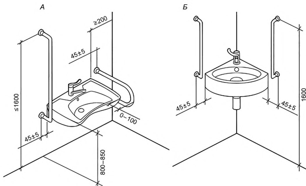
А — вариант установки поручней у раковины в стесненных условиях; Б — вариант установки поручней с угловой раковиной в стесненных условиях
