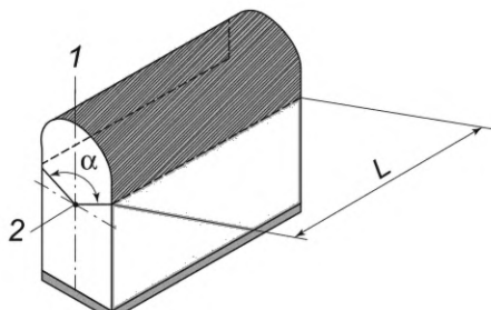
б) Симметричный без нечувствительной поверхности на концах
