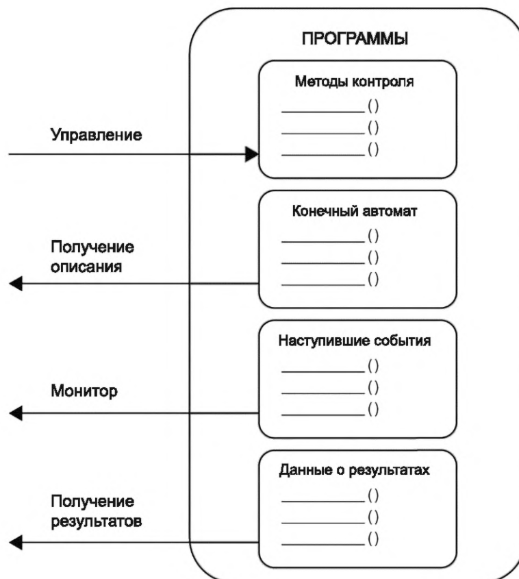
Рисунок 2 — Иллюстрация программы
