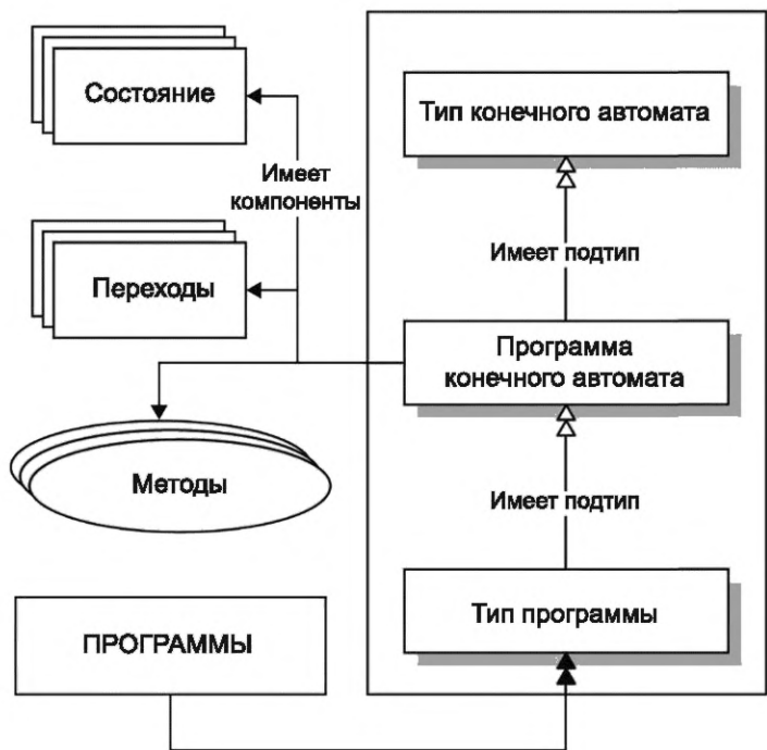
Рисунок 4 — Тип программы
