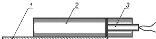
1 — пластина «свидетель»; 2 — заряд; 3 — электродетонатор
