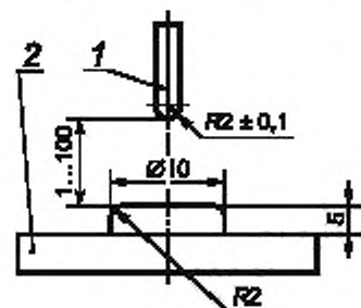
1, 2 — разрядные электроды из латуни
