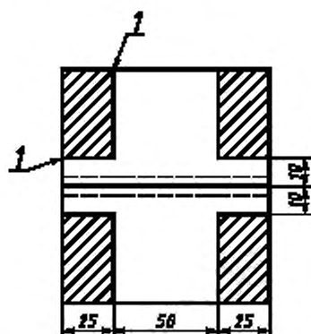
1 — линия разреза
