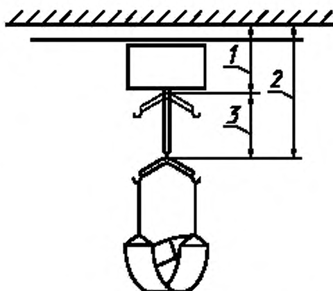
1 — верхнее положение системы опоры тела; 2 — нижнее положение системы опоры тела; 3 — рабочая зона подъемника
