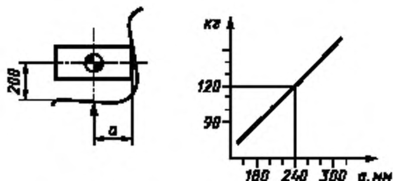
Рисунок 8 — Расположение нагрузки на жестком сиденье
