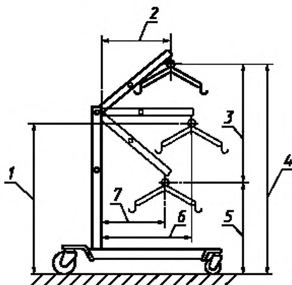
1 — высота системы опоры тела при максимальной дальности действия подъемника; 2 — дальность действия подъемника при верхнем положении системы опоры тела; 3 — рабочая зона подъемника; 4 — верхнее положение системы опоры тела; 5 — нижнее положение системы опоры тела; 6 — максимальная дальность действия подъемника; 7 — дальность действия подъемника при нижнем положении системы опоры тела
