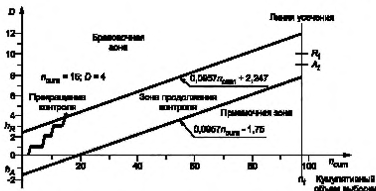
Рисунок 2 — Приемочная карта последовательного выборочного плана, рассматриваемого в примере пункта 2.4.3.2
