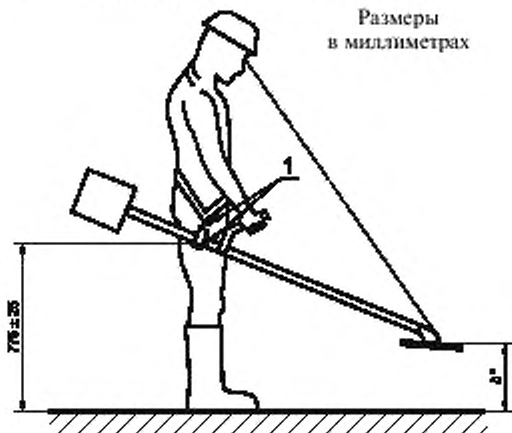
Рисунок 2 — Положение машины при испытании
