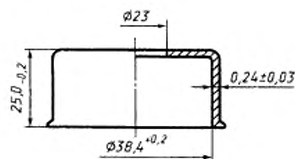
Рисунок 5 — Колпачок алюминиевый с накатываемой резьбой и центральным отверстием в дне 14А38
