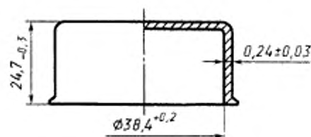
Рисунок 6 — Колпачок алюминиевый с накатываемой резьбой без отверстия в дне 14Б38
