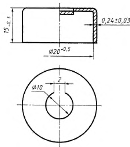
Рисунок 7 — Колпачок алюминиевый с накатываемой резьбой, надрезами на дне и лепестком для оттиба 14В20
