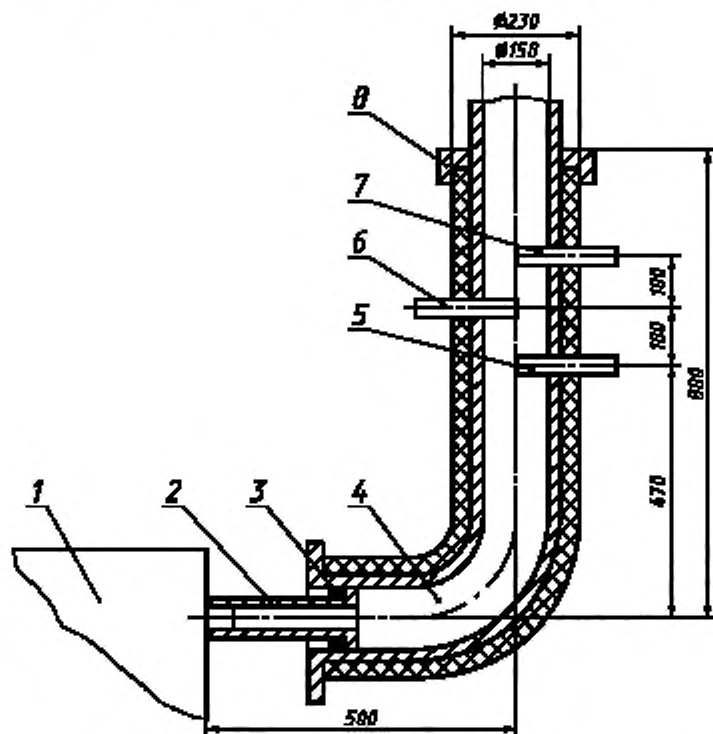
1 — аппарат; 2 — переходник; 3 — уплотнитель; 4 — труба; 5 — пробоотборник; 6 — термометр; 7 — трубка для измерения разрежения; 8 — крышка
