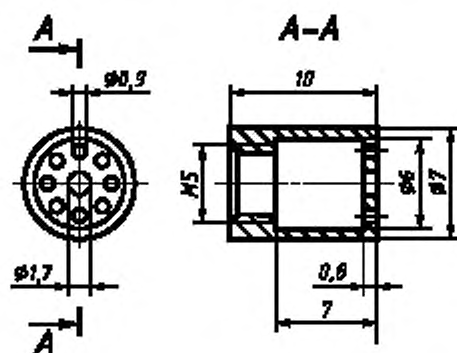
Рисунок Б.4 — Стабилизатор пламени
