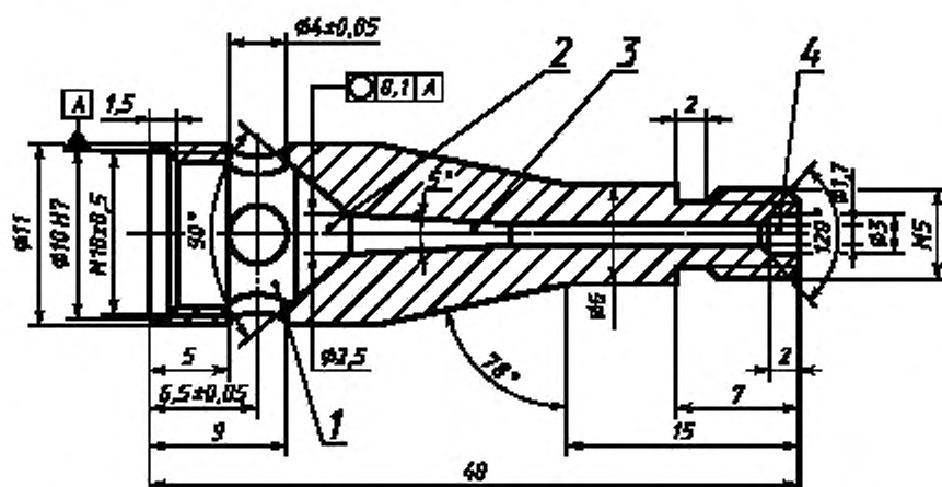
Рисунок Б.3 — Трубка горелки
